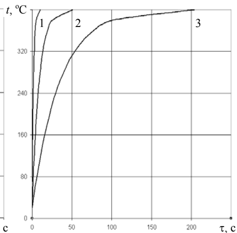
Рис. 4. Залежність t зразка з алюмінію від часу нагріву ( t печі 400^{\circ}\text{C} ): 1 – зразок d=0,005 м, l=0,02 м; 2 - d=0,01 м, l=0,05 м; 3 - d=0,02 м, l=0,1 м.
