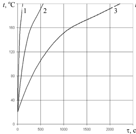
Рис. 1. Залежність t зразка зі сталі від часу нагріву ( t печі 200^{\circ}\text{C} ): 1 – зразок d=0,005 м, l=0,02 м; 2 - d=0,01 м, l=0,05 м; 3 - d=0,02 м, l=0,1 м.
