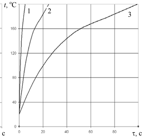
Рис. 2. Залежність t зразка з алюмінію від часу нагріву ( t печі 200^{\circ}\text{C} ): 1 – зразок d=0,005 м, l=0,02 м; 2 - d=0,01 м, l=0,05 м; 3 - d=0,02 м, l=0,1 м.
