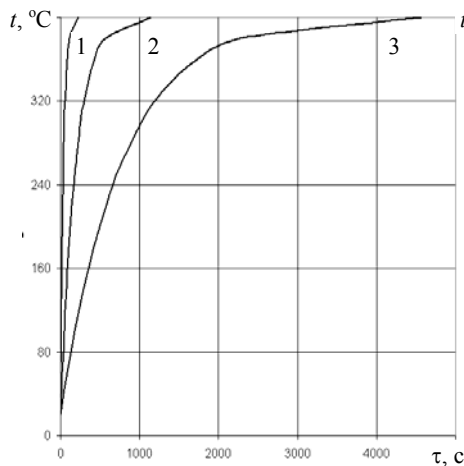
Рис. 3. Залежність t зразка зі сталі від часу нагріву ( t печі 400^{\circ}\text{C} ): 1 – зразок d=0,005 м, l=0,02 м; 2 - d=0,01 м, l=0,05 м; 3 - d=0,02 м, l=0,1 м.
