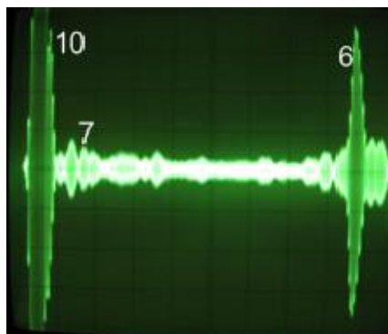
Рис. 2. Развертка на экране осциллографа при отсутствии дефектов на поверхности листа из стали ст.3 толщиной 30 мм длиной 1000мм.
