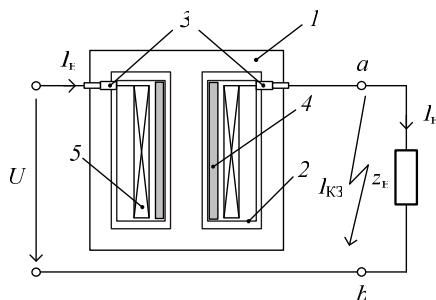
Рис. – Схематичне зображення НП обмежувача струму КЗ з екраном.
