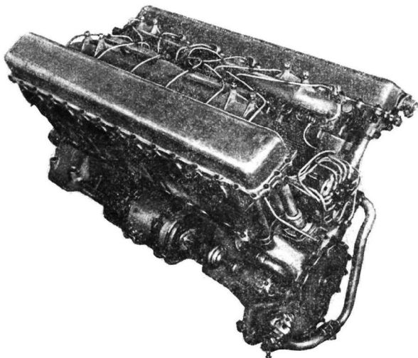
Рис. 1. Дизель БД-2, первенец танкового дизелестроения [4]
