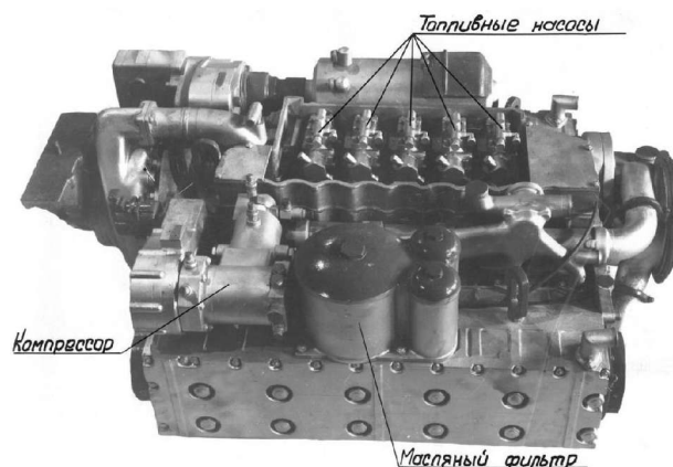
Рис. 4. Макет дизеля 5ТД – первого представителя второго поколения танковых дизелей
