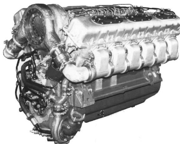
Рис. 3. Дизель В-92С2
