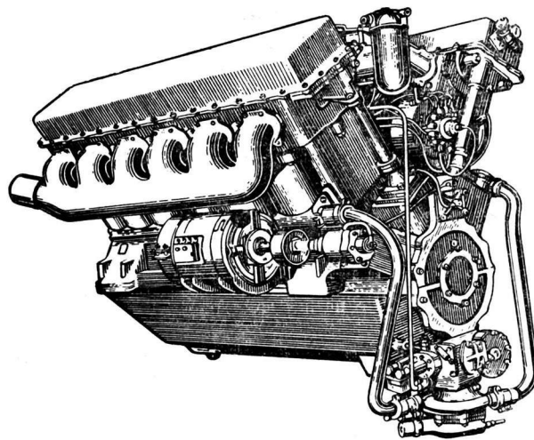
Рис. 2. Дизель В-2 [4]
