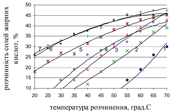
Рис. 2 – Залежність граничної розчинності мил пальмового стеарину (1), пальмової (2), кокосової (3), пальмоядрової (4) олій, пальмового олеїну (5), соняшnikової (6) і соєвої (7) олій в основі нейтралізуючого розчину від температури
