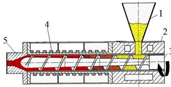
Рис. 1 – Схема вузла пресування шнекового гранулятора-екструдера: 1 – бункер; 2 – циліндр; 3 – шнек; 4 – нагрівач; 5 – формуюча головка.
