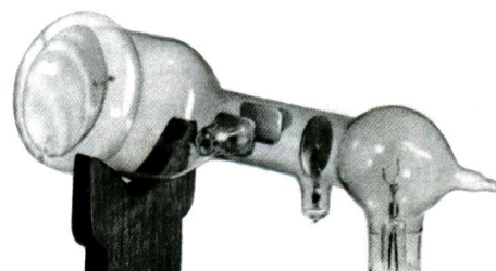
Рис. 26. Первая ЭЛТ конца 19-го века [3]
