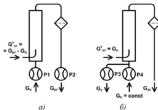
Рис. 2. Принципиальные схемы способов измерения G_{ог}^T :
