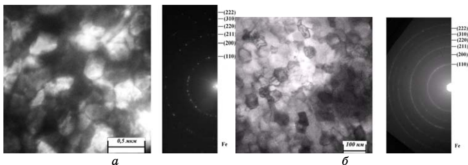
Рис. 1. Структура вакуумных конденсатов в исходном состоянии: a — Fe ( T_p 250°C); б — Fe-W ( T_p 250°C, W \cong 0,8 ат.%).
