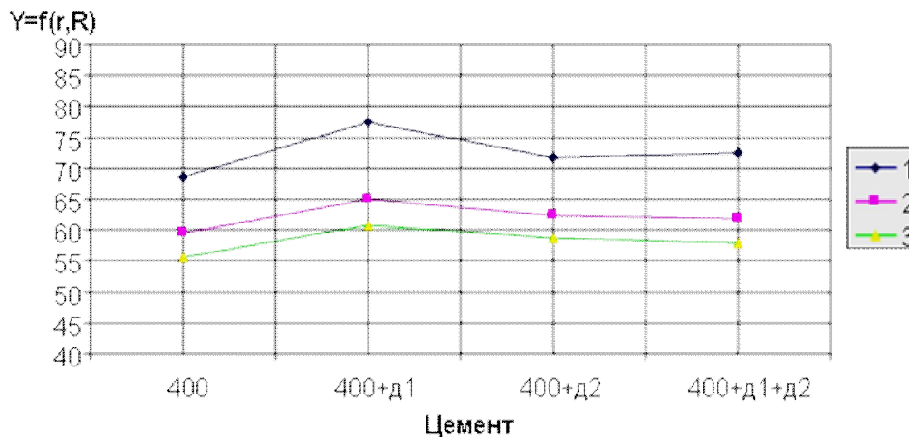
Рис. – Графические зависимости для определения приведенной активности цемента с добавками по результатам испытаний стандартных балочек на изгиб (r) и сжатие (R):
