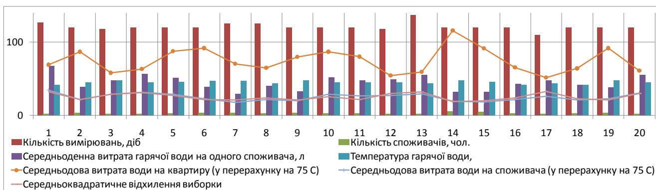
Рисунок 2 – Дані вимірювань витрати гарячої води
