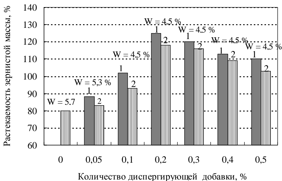
Рис. 2. Зависимость растекаемости при вибрации в течение 30 секунд крупнозернистой корундовой с добавкой \text{Cr}_2\text{O}_3 массы от количества вводимой диспергирующей добавки
