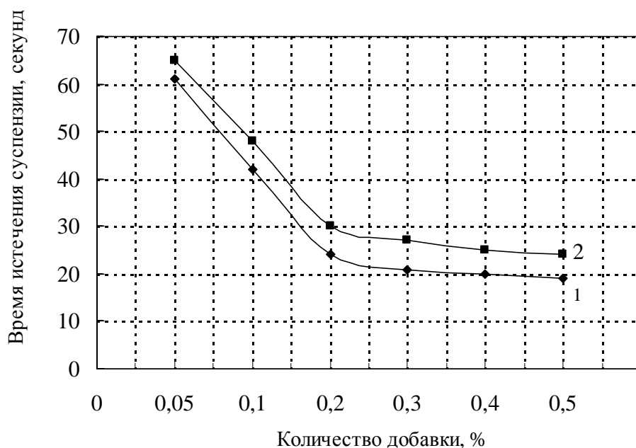
Рис. 1. Зависимость времени истечения суспензии от количества вводимой диспергирующей добавки:
