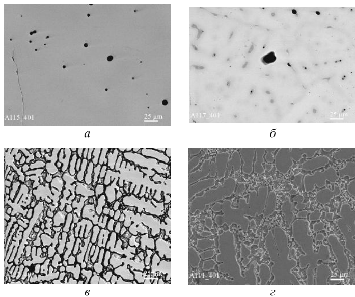
Рис. 1 – Микроструктура сплава на основе системы Nb-Cr-Ti-Zr-Al: а, б – нетравленная поверхность; в, г – травленные шлифы
