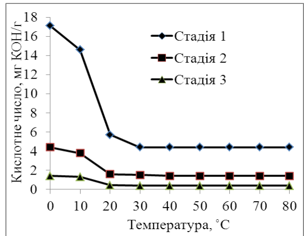
Рисунок 3 – Залежність кислотного числа від температури екстракційної рафінації ЖКО
