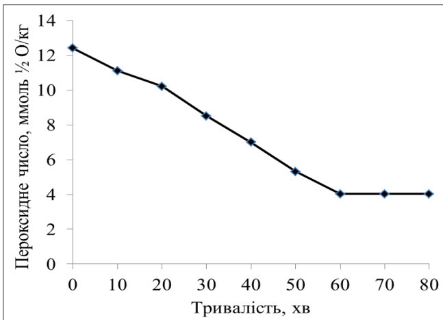
Рисунок 4 – Залежність пероксидного числа від тривалості екстракційної рафінації ЖКО (КЧ=0,38 мг КОН/г) при співвідношенні ЖКО:етанол 1:4 та t=78^{\circ}\text{C}
