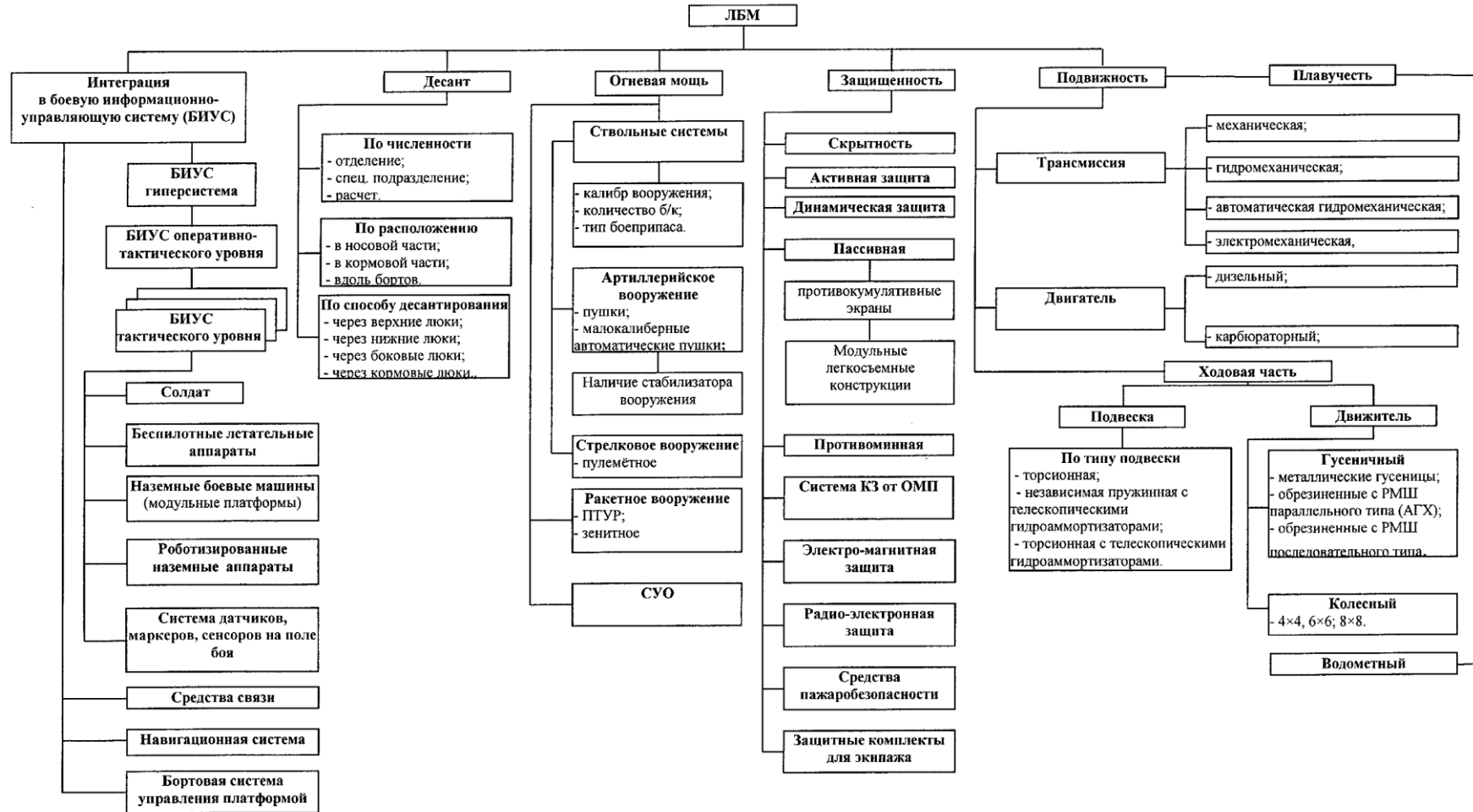
Рисунок 1 – Классификация легких колёсных и гусеничных боевых бронированных машин
