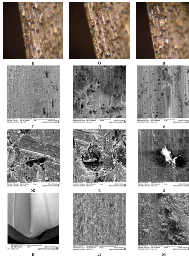
Рисунок 5 – Характер и морфология рабочих поверхностей алмазных кругов после обработки хрустала - круг № 1 (а, г, ж), круг № 2 (б, д, з), круг № 5 (в, е, и); вид обработанной поверхности хрустала (к, л, м)
