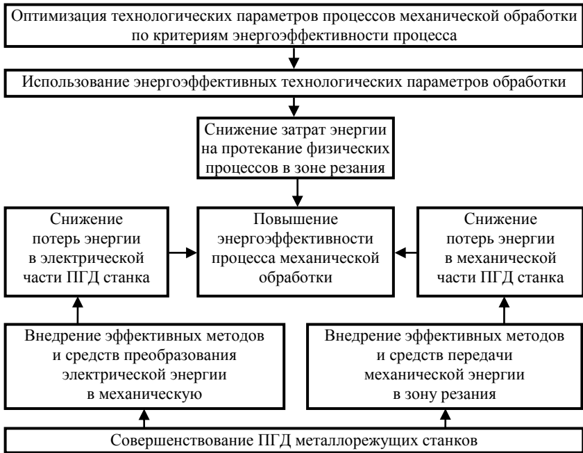
Рисунок 1 – Направления повышения энергоэффективности процессов механической обработки деталей на тяжелых токарных станках
