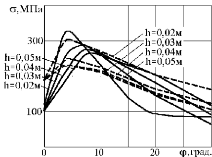
Рисунок 7 – Максимальные напряжения \sigma_x в колесном центре без бандажа при его нагреве под посадку на ось в момент окончания нагрева: — — зона перелома ступицы в диск, - - - зона перелома дисковой части в бандаж (вент)
