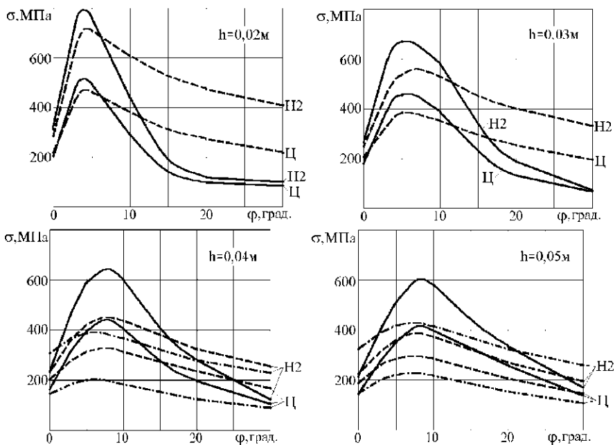
Рисунок 5 – Максимальные напряжения \sigma_c в собранной модели при нагреве ступицы под посадку на ось в момент окончания нагрева: — — зона перехода ступицы в диск, — — зона перехода ступицы в бандаж (венец); — — зона контакта центра и бандажа
