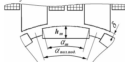
Рис. 3 Фрагмент поперечного перетину ВД
