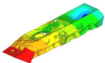
Полные перемещения: выстрел на борт
