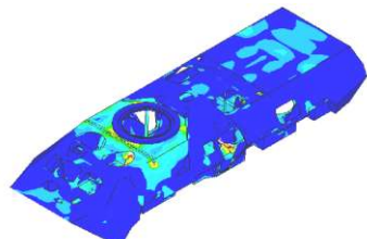
Эквивалентные напряжения по Мизесу: выстрел по курсу
