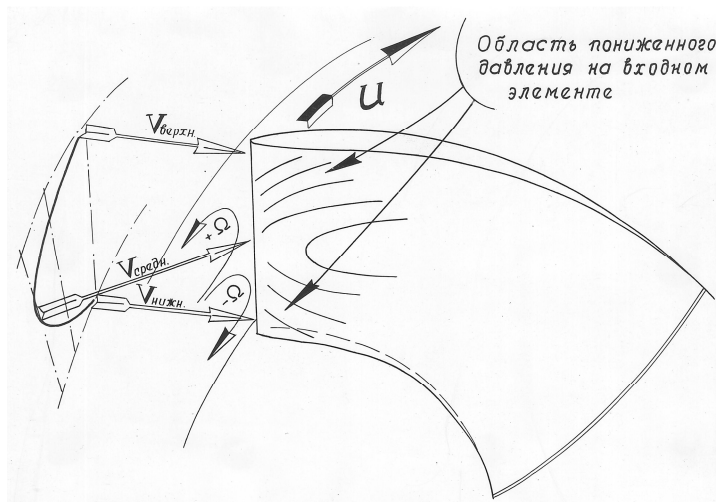
Рис. 12 – Форма натекающего потока на входе в рабочее колесо
