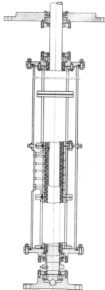
Рис. 9 – Съемник давления (разрез)
