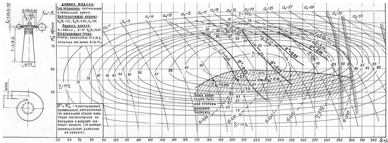
Рис. 13 – Зоны возникновения начальной кавитации на поверхностях лопастей
