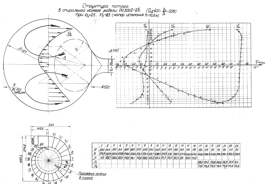
Рис. 4 – Структура потока в спиральной камере
