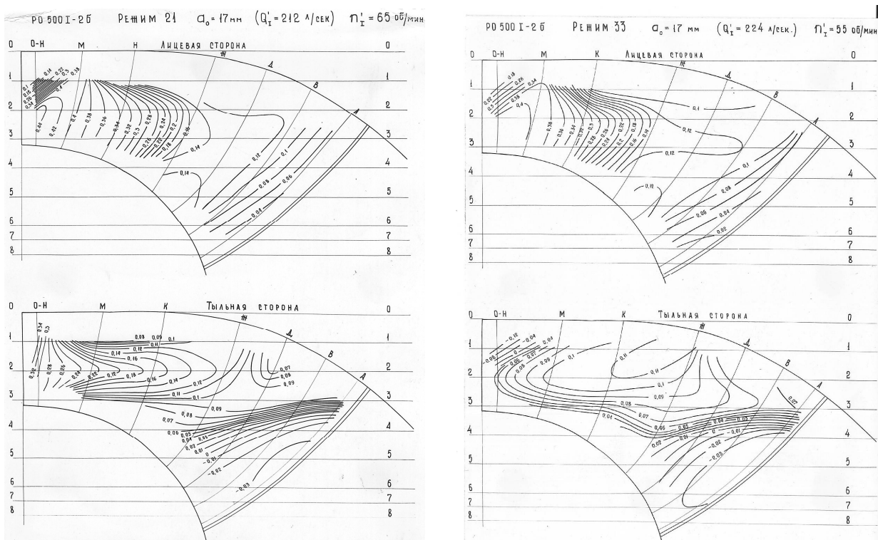
Рис. 11 – Изолинии равного давления на лицевой и тыльной стороне лопасти на различных режимах
