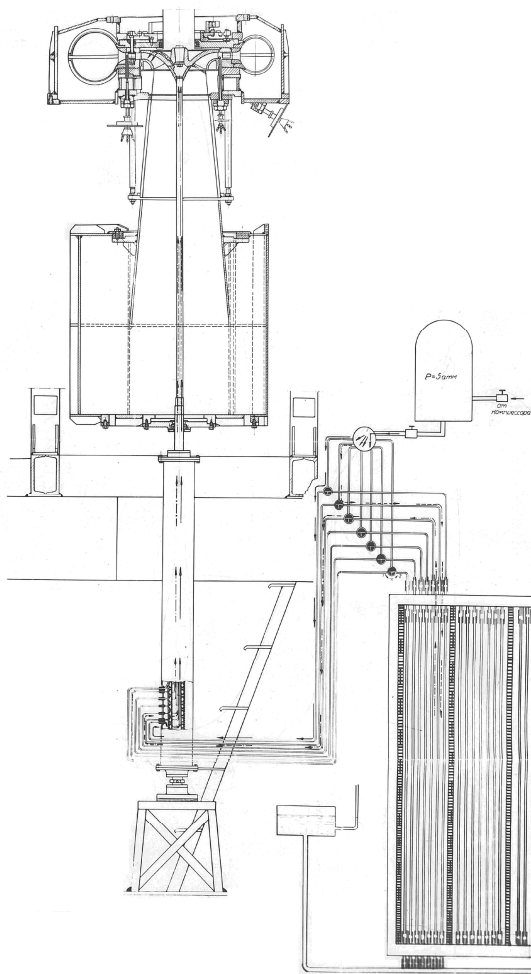
Рис. 8 – Устройство для опытного определения распределения давления на вращающихся лопастях гидромашин
