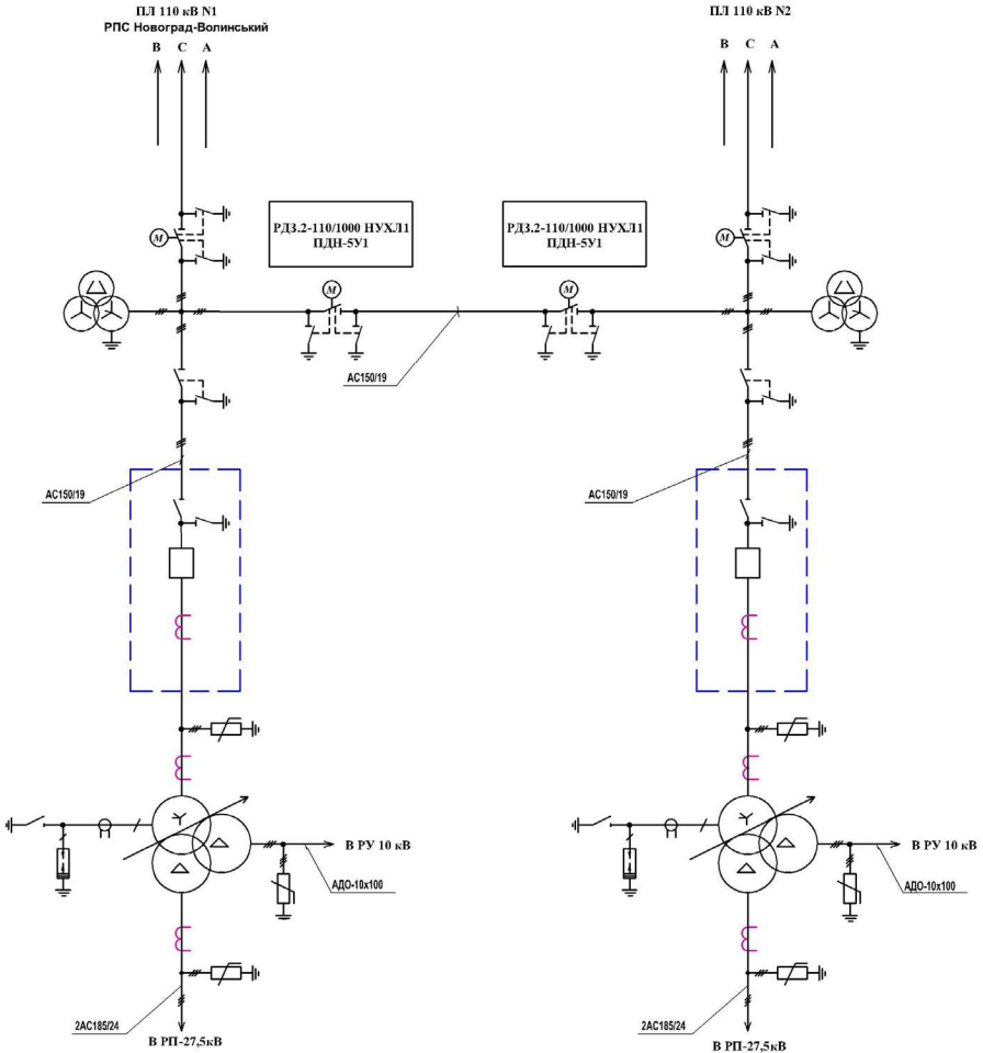
Рис. 4 – Рекомендована схема головних електричних з'єднань отпаечної тягової підстанції 220 – 110 кВ
