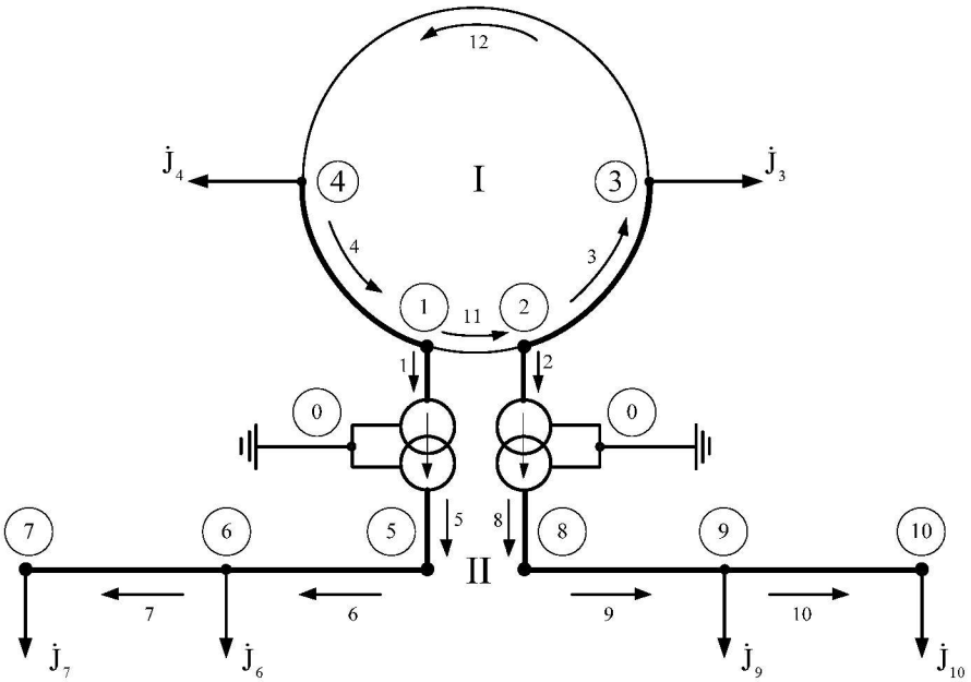
Рис. 5 – Схема зовнішнього і тягового електропостачання:
