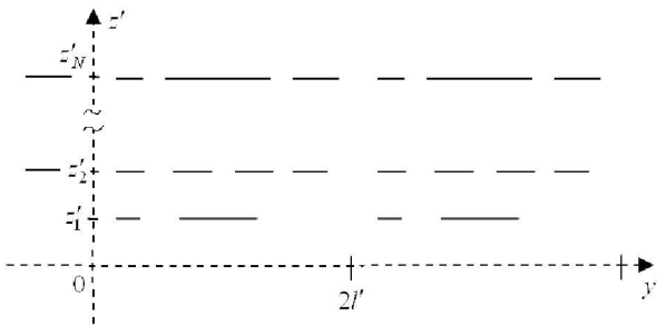
Рис. 1 – Сечение дифракционной структуры плоскостью Y'OZ' .
