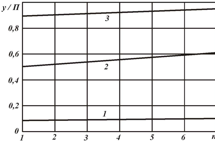
Рис. 2 – Залежність відносної величини y/\Pi від кількості проходів круга n : 1 – B_{1_{баз}} = 0,1 ; 2 – B_{1_{баз}} = 1 ; 3 – B_{1_{баз}} = 10 .
