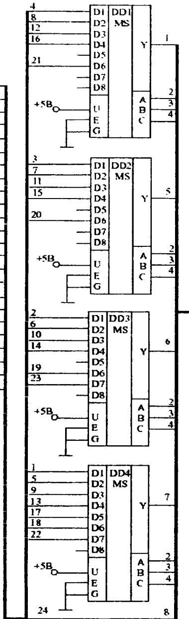
Рис. Принципиальная электрическая схема устройства сопряжения
