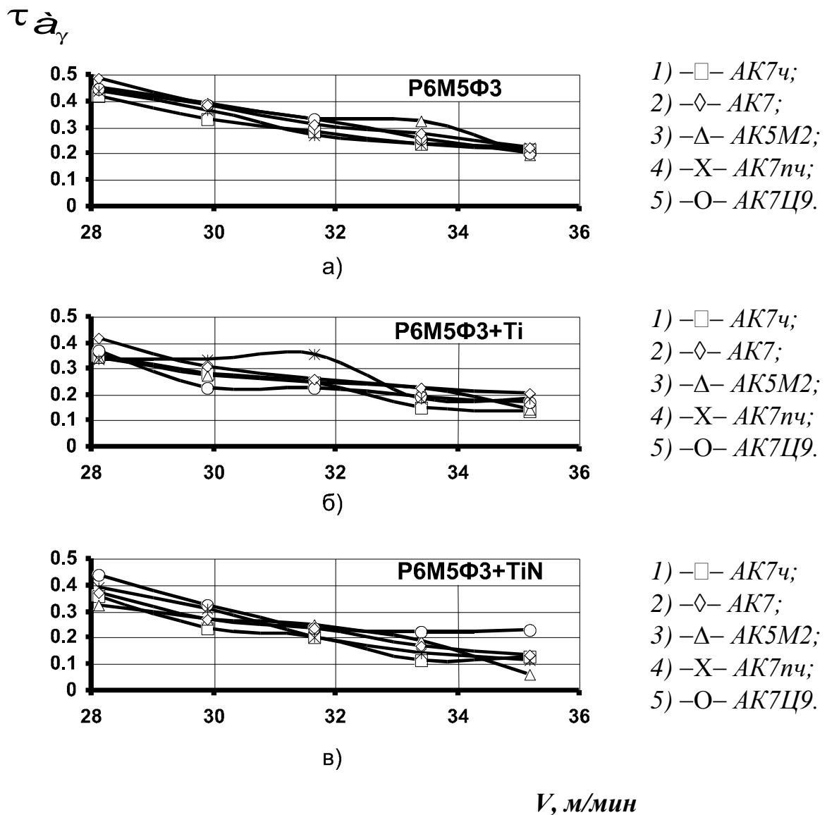
Рис. 4 – Влияние скорости резания V, \text{ м/мин} на адгезионную составляющую суммарной удельной силы трения \Delta\tau_{a\gamma} , МПа на поверхности A\gamma , при взаимодействии стали P6M5Φ3, износостойких покрытий КОН Ti 6 изн. и КОН TiN 10 изн с алюминиями.
