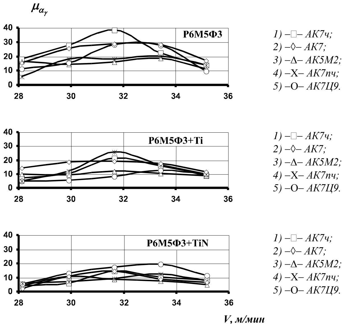
Рис. 3 – Влияние скорости резания V , м/мин на адгезионную составляющую коэффициента трения \mu_{\alpha\gamma} на поверхности A\gamma при взаимодействии стали Р6М5Φ3, износостойких покрытий КОН Ti 6 изн. и КОН TiN 10 изн. с алюминия.
