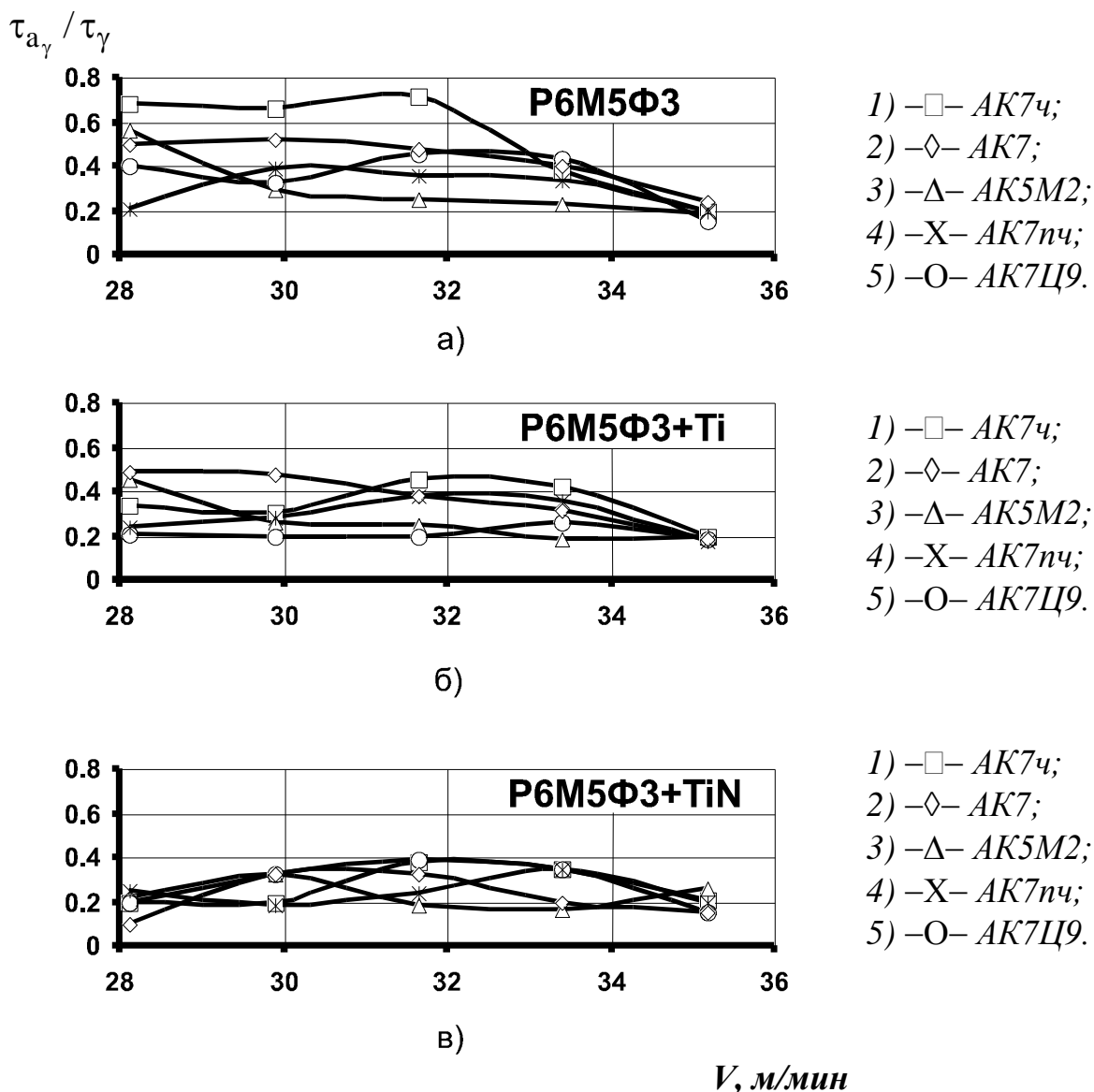
Рис. 5 – Влияние скорости резания V, \text{ м/мин} на отношение адгезионной составляющей к суммарной удельной силы трения \tau_{a\gamma} / \tau_{\gamma} на поверхности A\gamma , при взаимодействии стали P6M5Φ3, износостойких покрытий КОН Ti 6 изн. и КОН TiN 10 изн. с ЛАС.
