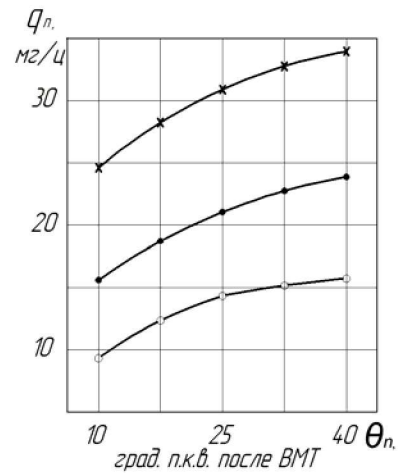
Рис. 5. Параметры предварительной порции топлива q_n^M : o – 1-сопловый распылитель; • – 4-сопловый распылитель; x – 5-сопловый распылитель
