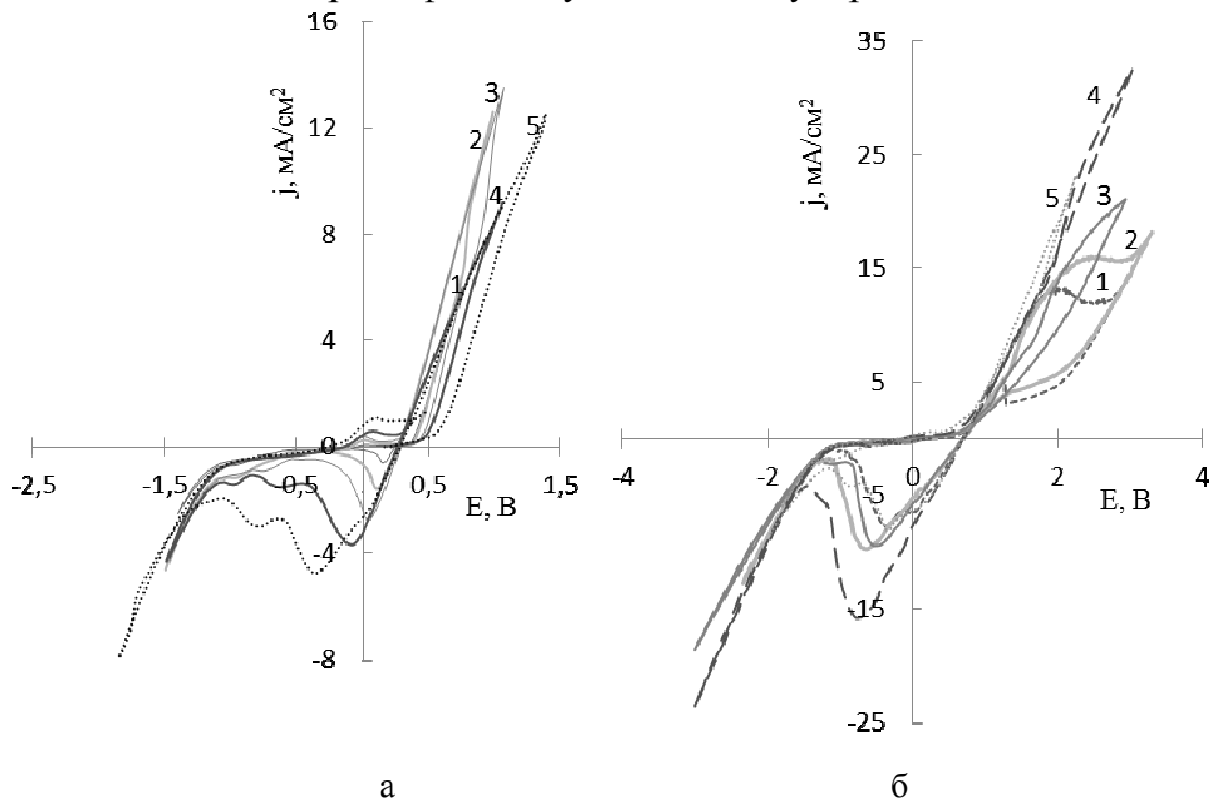
Рисунок 2 - Вольтамперограммы меди (а) и серебра (б) в водном растворе 0,1 N Na 2 SO 4 при скорости развертки потенциала, мВ/с: 1 – 5; 2 – 10; 3 – 20; 4 – 50; 5 – 100
