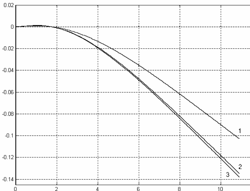
Рисунок 3 – Функция прогиба
