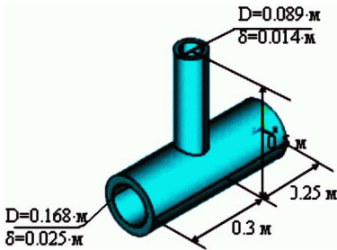
Рисунок 1 – Геометрія конструкції трійника
