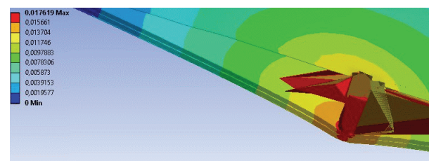
Рисунок 3 – Распределение перемещений в пластине с покрытием при скорости удара 100 м/с
