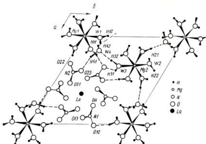
Рис. 6 – Структурний мотив кристалів [\text{Mg}(\text{H}_2\text{O})_6]_3[\text{Ln}(\text{NO}_3)_6]_2 \cdot 6\text{H}_2\text{O} ( \text{Ln} - \text{La} - \text{Sm} ) у проекції на площину ab
