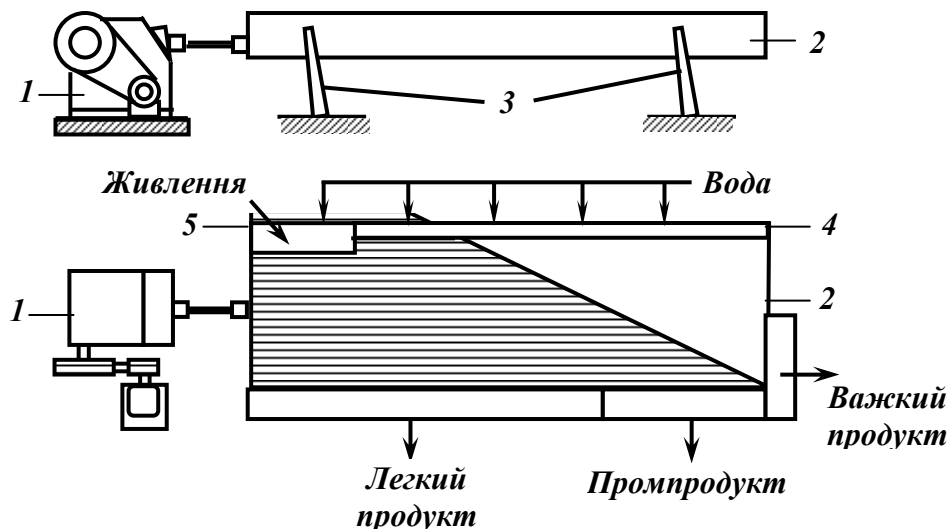
Рис. 5.31 – Схема концентраційного стола .
