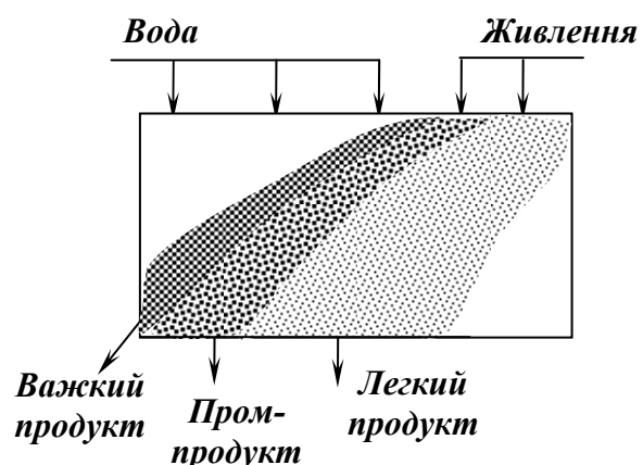
Рис. 5.34 – Схема розподілу продуктів на деці концентраційного столу ( \delta_{к-т} > \delta_{пн} > \delta_{відх} ).
