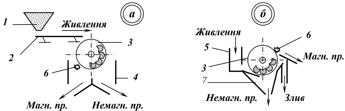
Рис. 7.8 – Схеми барабанних магнітних сепараторів.
