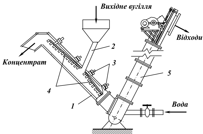
Рис. 5.39 – Крутопохилий сепаратор.
