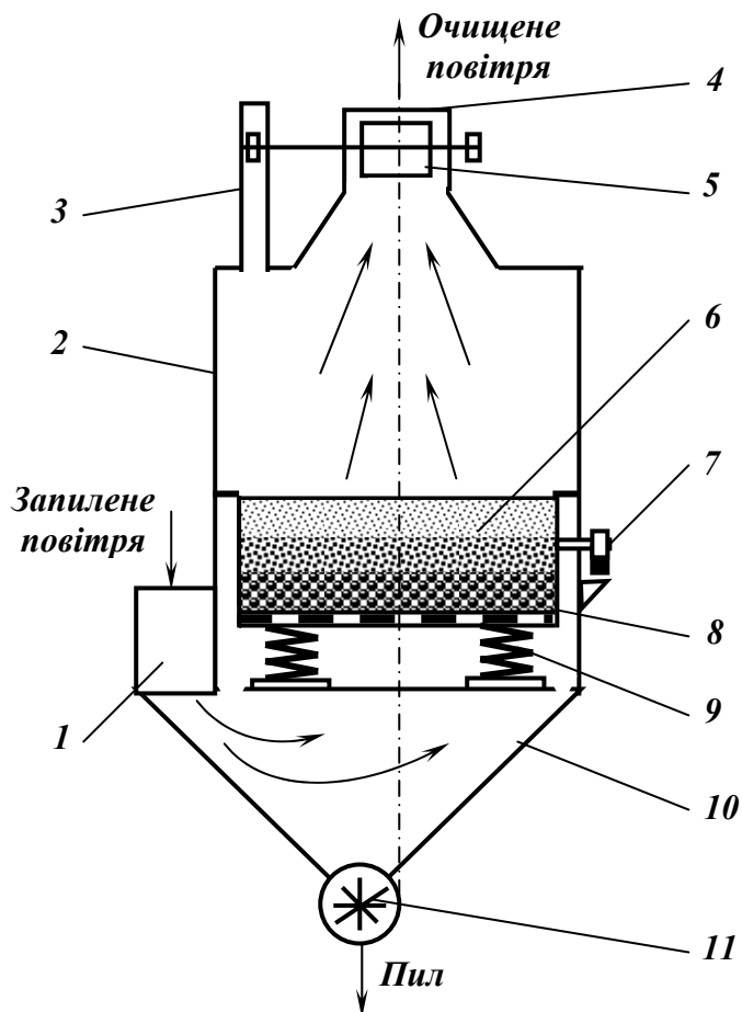
Рис. 10.35 – Зернистий фільтр з регенерацією методом зворотної продувки і накладення вібрацій.
