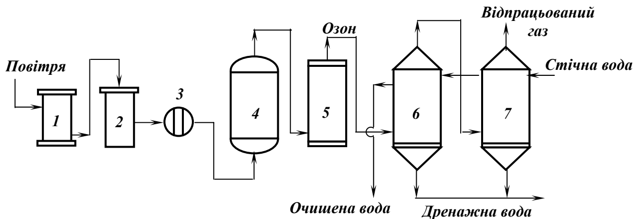
Рис. 12.2 – Схема озонаторного пристрою.
