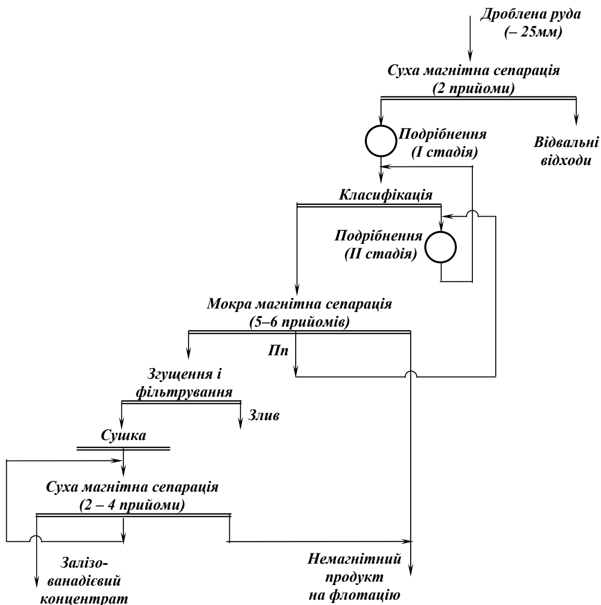
Рис. 7.18 – Схема магнітного збагачення титаномагнетитової руди.
