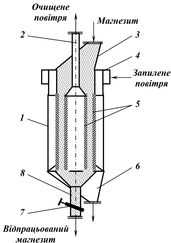
Рис. 10.34 – Зернистий фільтр з вертикальним пересувним шаром магнезиту.
