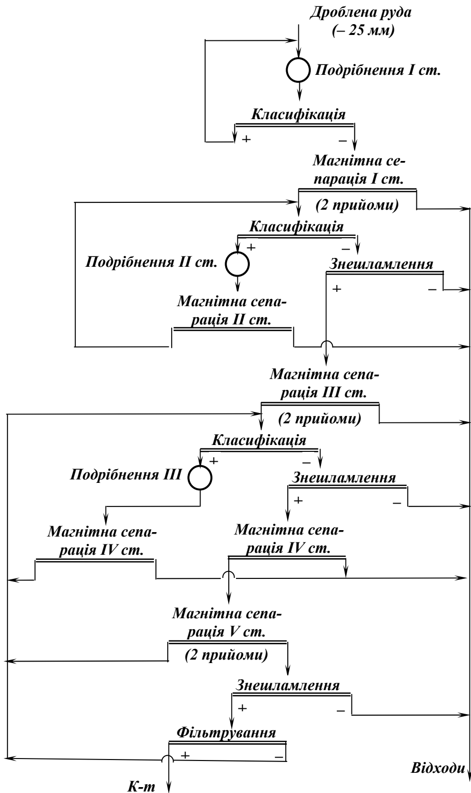
Рис. 7.17 – Схема мокрого магнітного збагачення тонковкраплених залізистих кварцитів.
