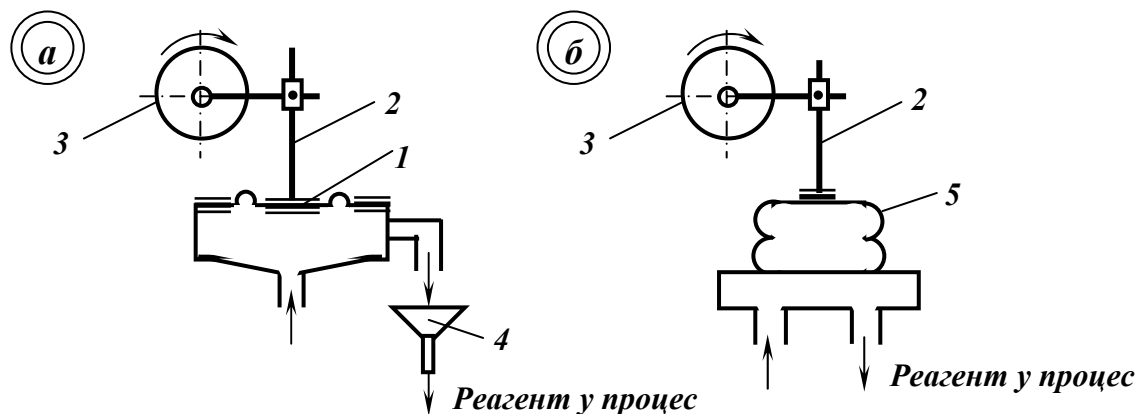
Рис. 6.23 – Схеми діафрагмового живильника і сифонного дозатора.
