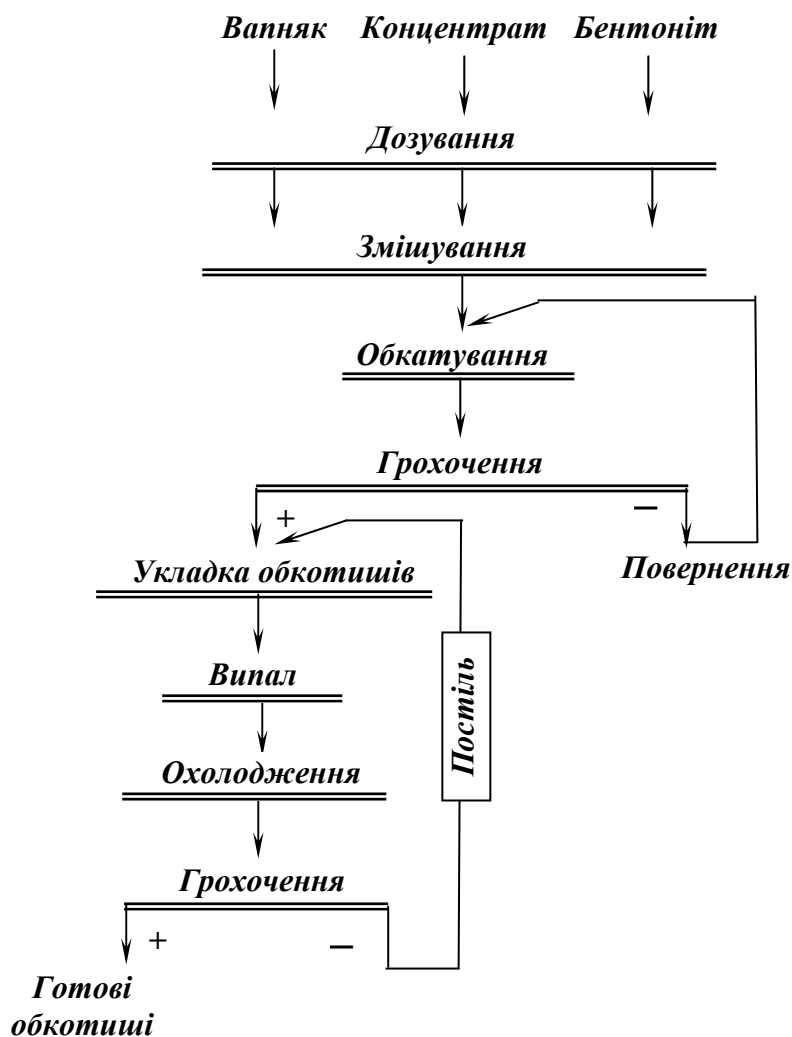
Рис.10.41 – Схема виробництва обкотишів (котунів).
