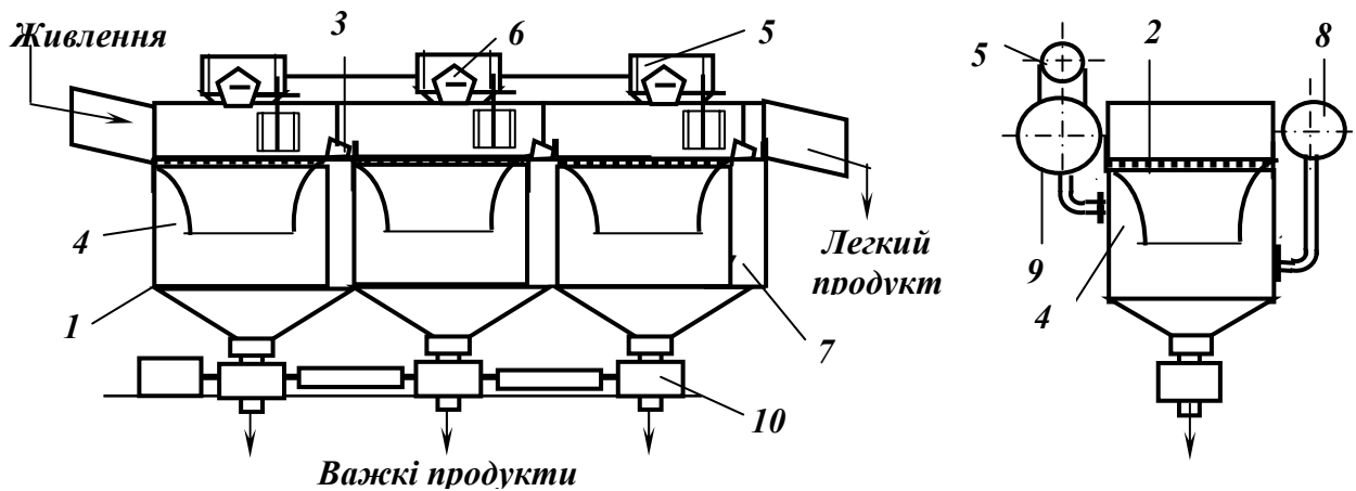
Рис. 5.22 – Схема відсаджувальної машини ОПС-13.
