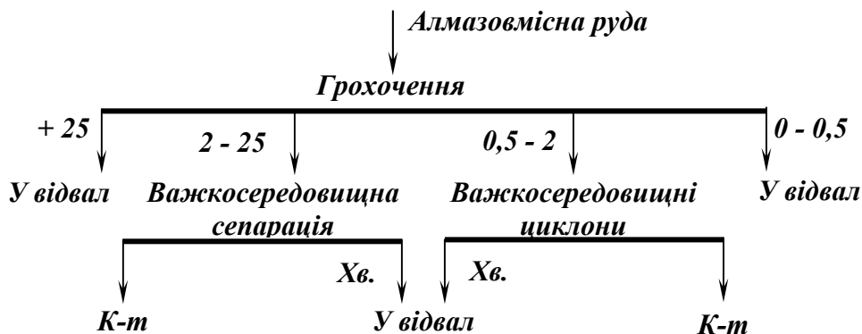
Рис. 5.16 – Схема важкосередовищного збагачення алмазовмісних розсіпів.
