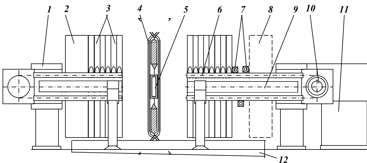
Рис. 10.17 – Схема фільтр-преса.
