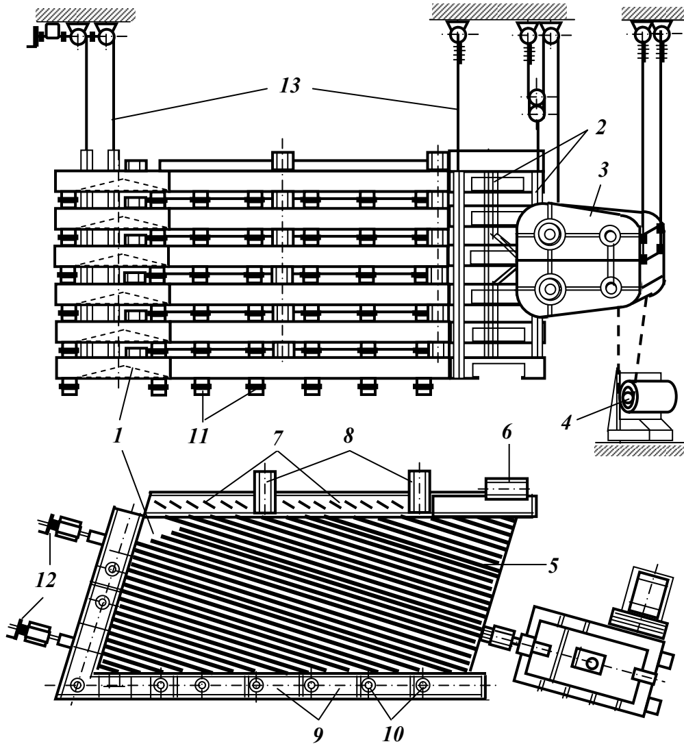
Рис. 5.37 - Схема концентраційного стола СКПМ-6.
