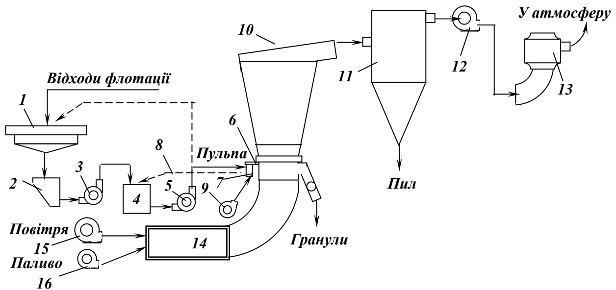
Рис. 11.12 – Схема технологічної установки для грануляції відходів флотації.
