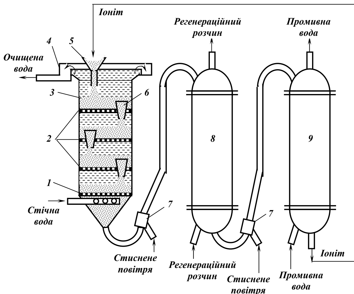
Рис. 12.3 – Схема йонообмінного пристрою.
