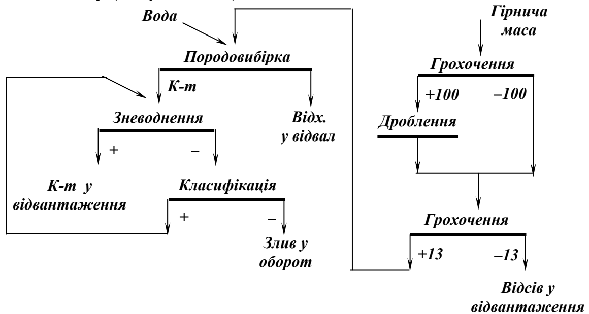
Рис. 5.42 – Схема механізованої породовибірки з використанням крутопохилого сепаратора.
