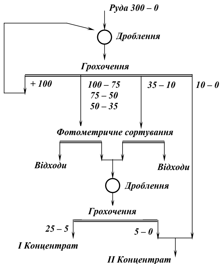
Рис. 9.19 – Технологічна схема фотометричного сортування доломітової руди.
