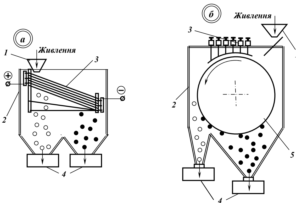
Рис. 8.10 – Діелектричні сепаратори.
