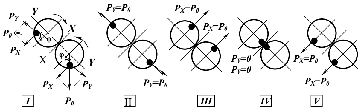
Рис. 4.16– Принцип дії самобалансного вібробудувача.
