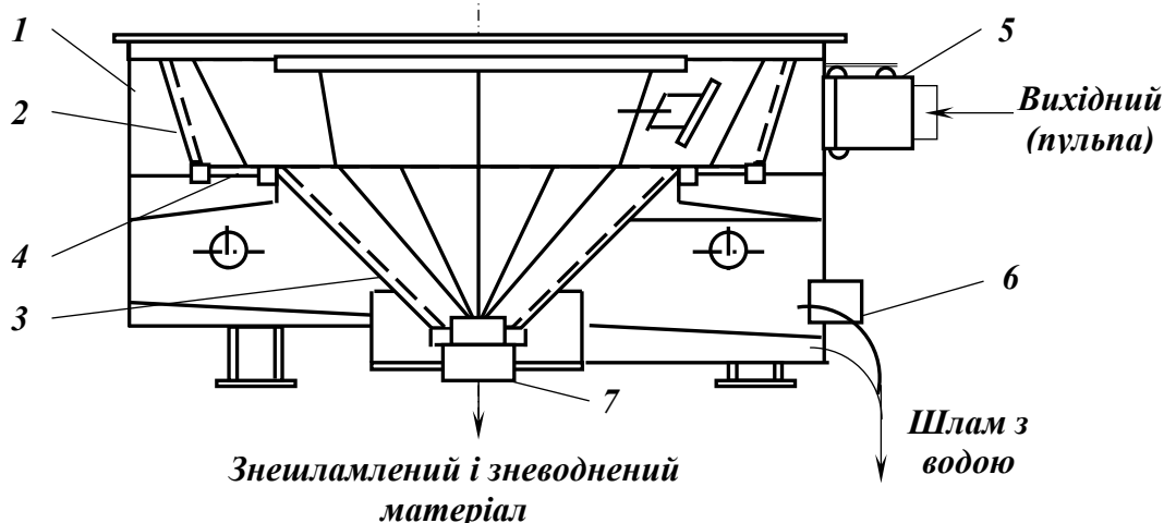
Рис. 4.8 – Конусний грохот.
