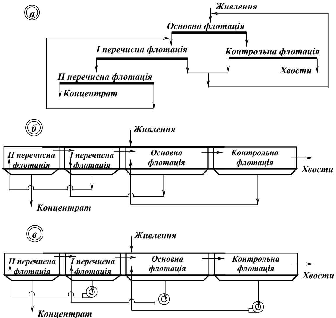
Рис. 6.13 – Розподіл операцій флотації схеми a по флотаційним машинам: б – механічним і пневмомеханічним; в – пневматичним.
