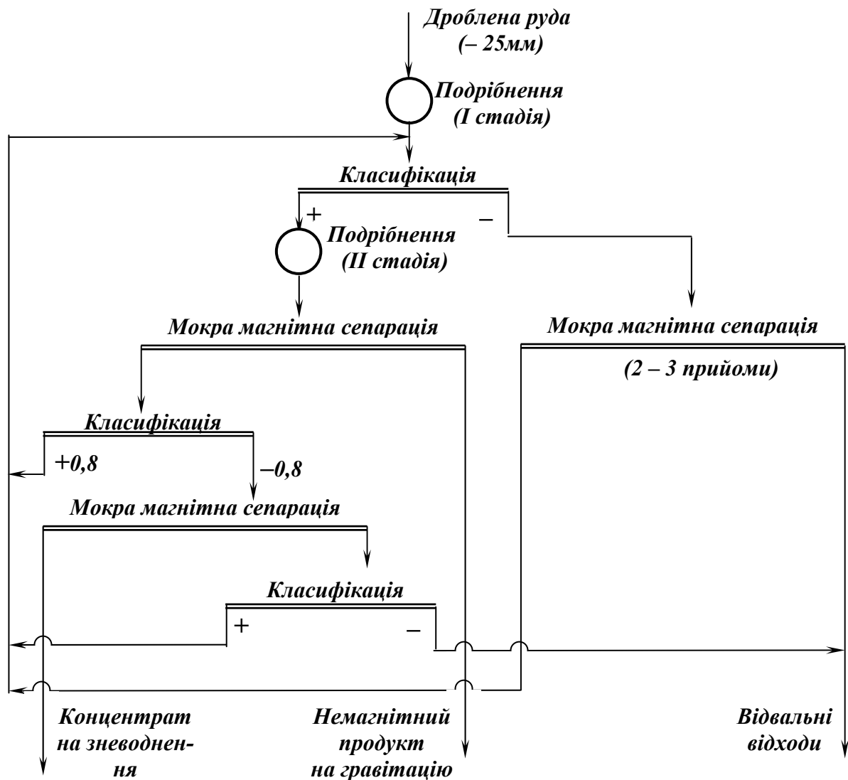
Рис. 7.19 – Схема мокрого магнітного збагачення дрібновократленої магнетито-гематитової руди.
