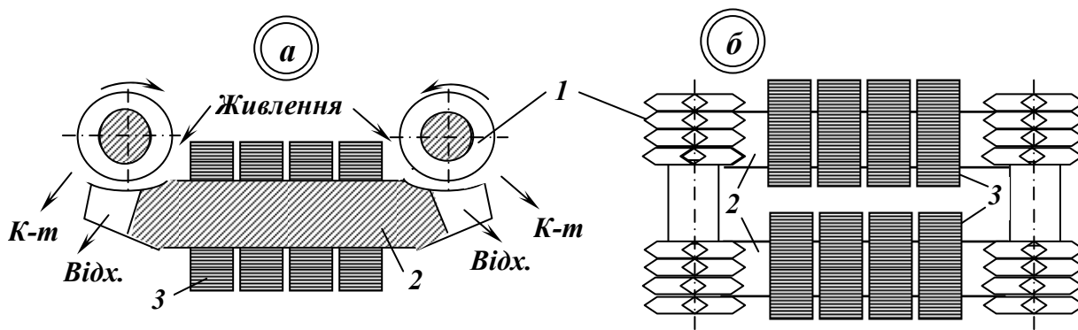
Рис. 7.11 – Схема валкового електромагнітного сепаратора.
