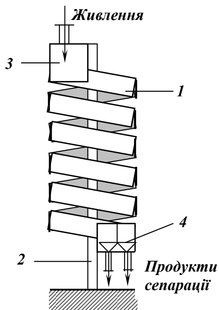
Рис.5.36 – Схема гвинтового сепаратора.
