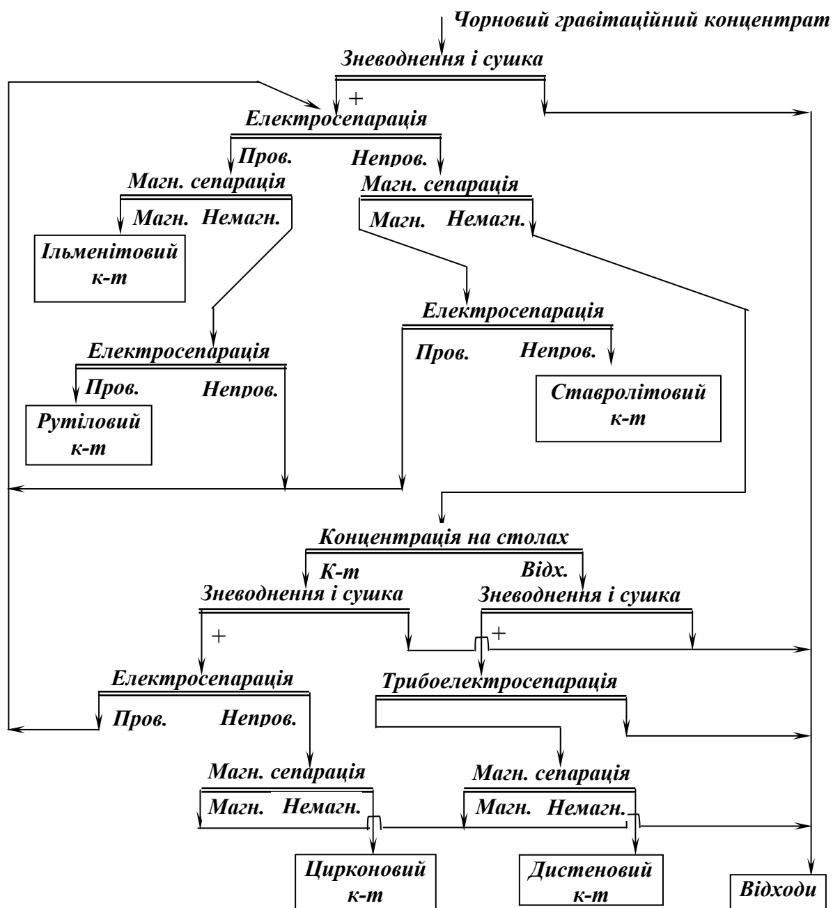
Рис. 8.11 – Схема доводки чорнових гравітаційних концентратів при збагаченні титано-цирконієвих розсіпних руд.
