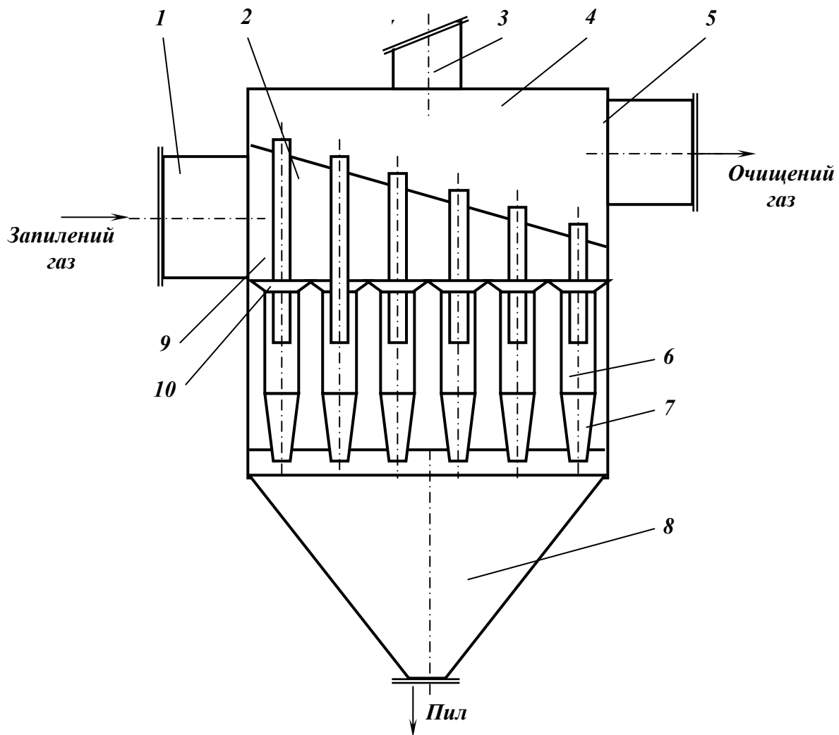
Рис. 10.29 – Схема батарейного циклона.
