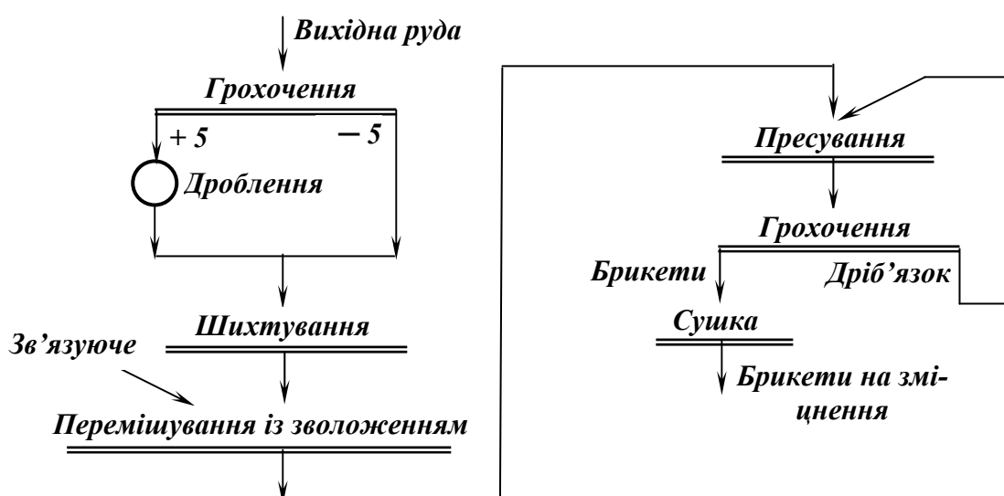
Рис.10.39 – Схема брикетування рудної сировини.
