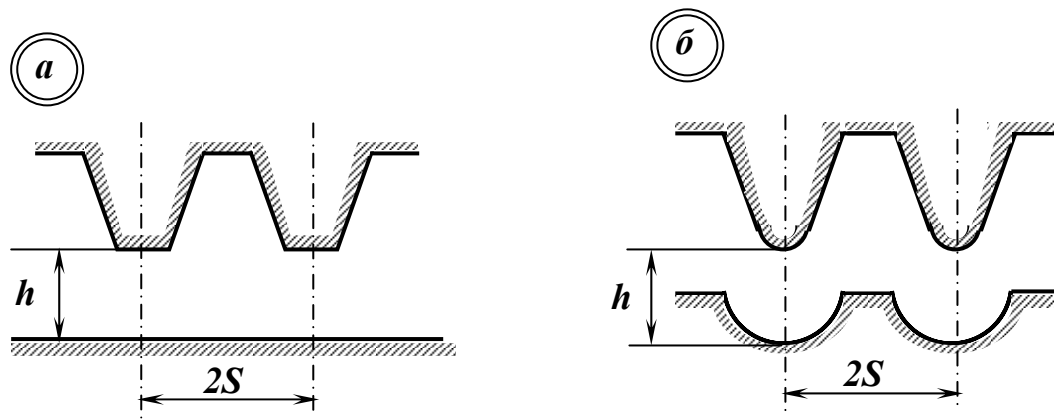
Рис. 7.7 – Профілі робочих зон сепараторів з сильним магнітним полем. a – трапецієподібний зубець – плоский полюс; б – закруглений зубець – жолобчатий полюс.
