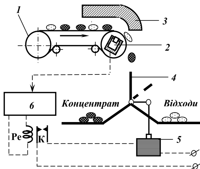
Рис. 9.11 – Схема стрічкового радіометричного сепаратора. 1 – конвеєр; 2 – датчик; 3 – екран; 4 – шибер; 5 – електромагніт; 6 – радіометр.
