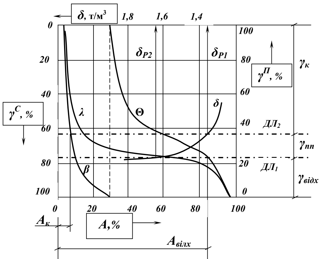
Рис. 5.2 – Криві збагачуваності вугілля.
