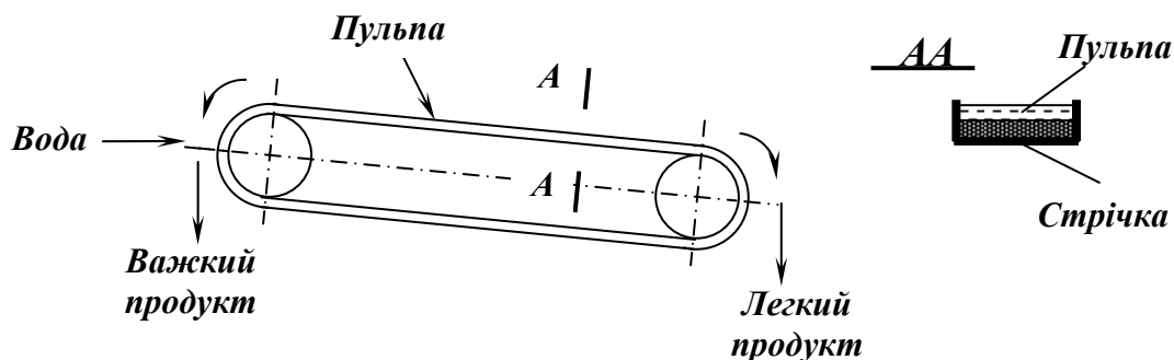
Рис. 5.29 – Схема шлюзу з рухомим уловлюючим покриттям.
