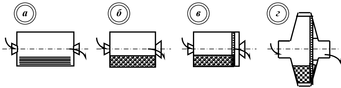
Рис. 4.39 – Схеми барабаних млинів: a – стержневий млин МСЦ; б – кульовий млин МШЦ; в – кульовий МШР або рудногальковий МРГ млини; z – млин мокрого самоподрібнення.
