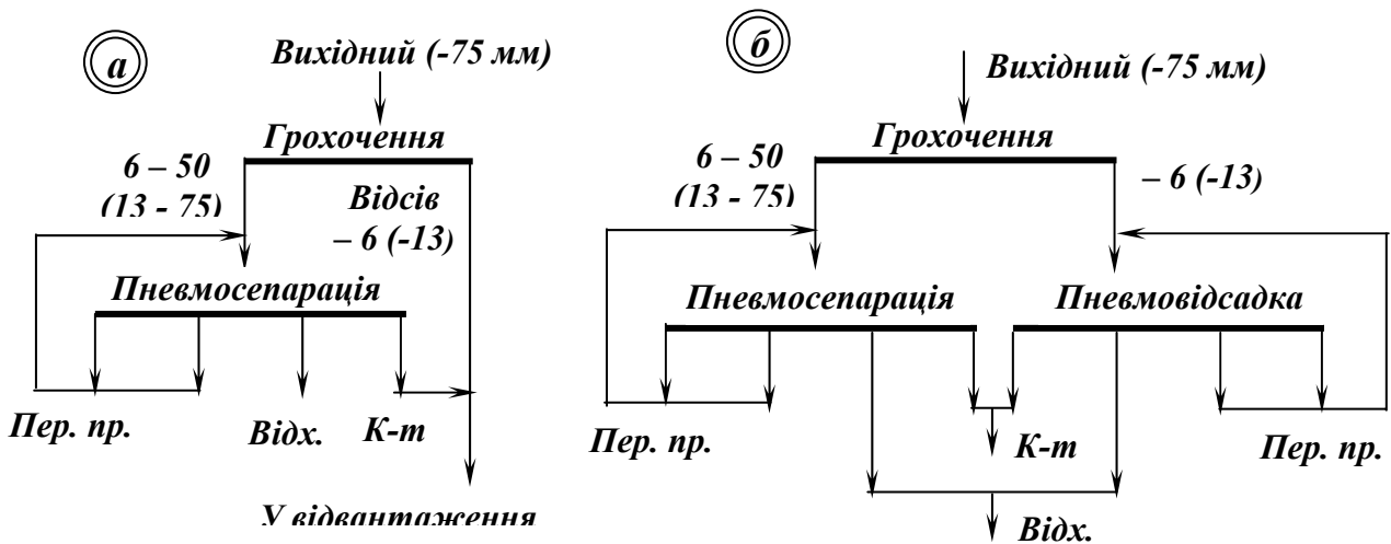
Рис. 5.51 – Схеми пневмозбагачення вугілля. a – глибина збагачення 6 (13) мм; б – глибина збагачення 0 мм.
