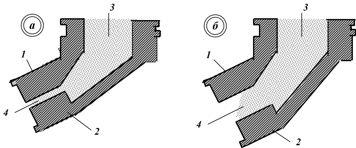
Рис. 4.29 – Схема процесу в камері дроблення дробарки «Жиродиск». а – чаша і конус-диск зближені – матеріал дробиться; б – вихідна щілина розкрита – матеріал розвантажується; 1 – футеровка чаші; 2 – футеровка конуса-диска; 3 – камера дроблення; 4 – паралельна зона дробарки.
