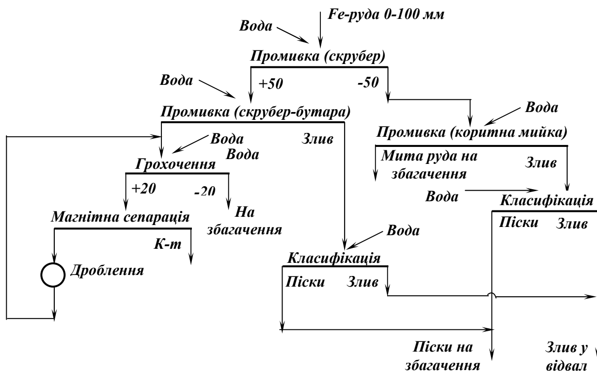
Рис. 4.50 – Схема промивки важкопромивної залізної руди.
