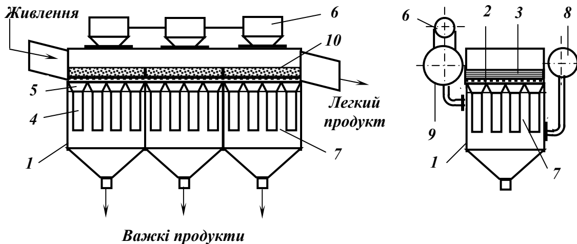
Рис. 5.19 – Схема відсаджувальної машини ОПМ-13.
