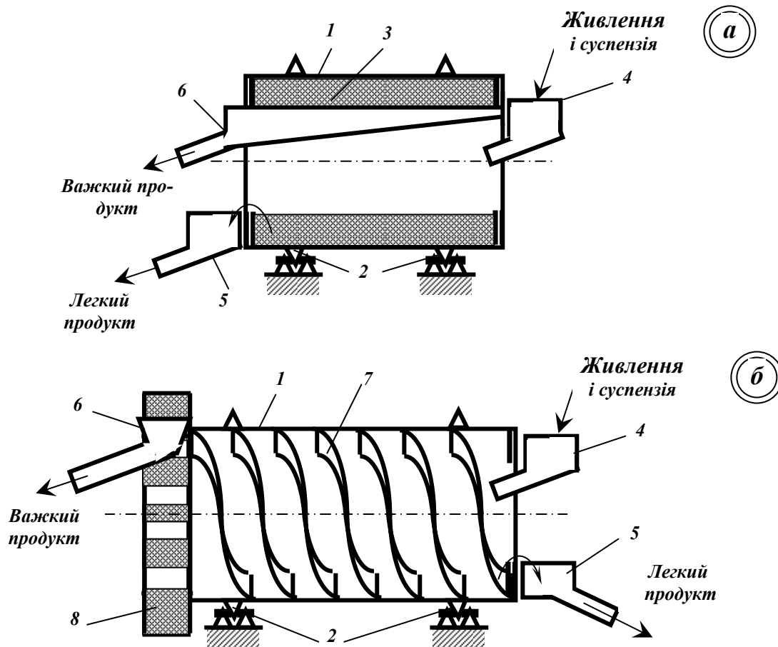
Рис. 5.7 – Схеми барабанних важкосередовищних сепараторів: а – елеваторний сепаратор СБЕ; б – спіральний сепаратор СБС. 1 – барабан; 2 – опорні катки; 3 – перфоровані лопаті; 4 – завантажувальний жолоб; 5 – розвантажувальний жолоб легкого продукту; 6 – розвантажувальний жолоб важкого продукту; 7 – двозахідна спіраль; 8 – лопатний елеватор.
