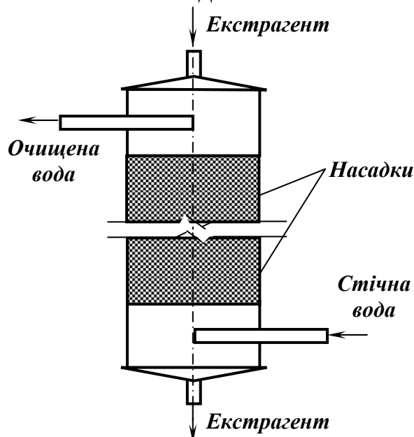
Рис. 12.4 – Екстракційна колона.
