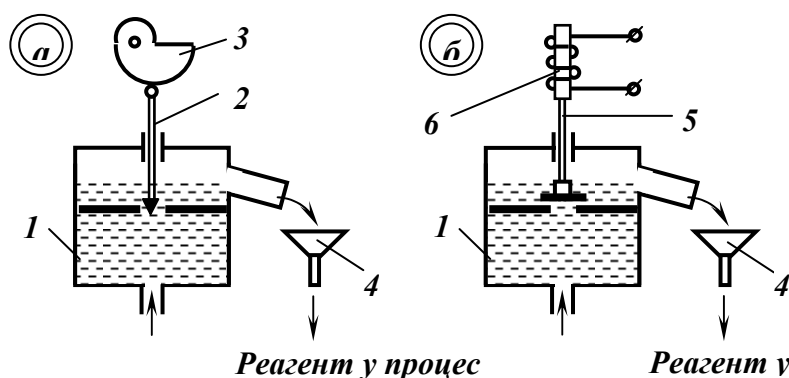
Рис. 6.21 – Схеми голчатого і клапанного живильників.
