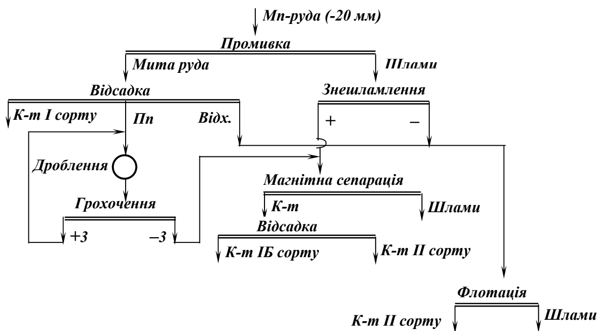
Рис. 7.22 – Схема збагачення оксидної марганцевої руди.
