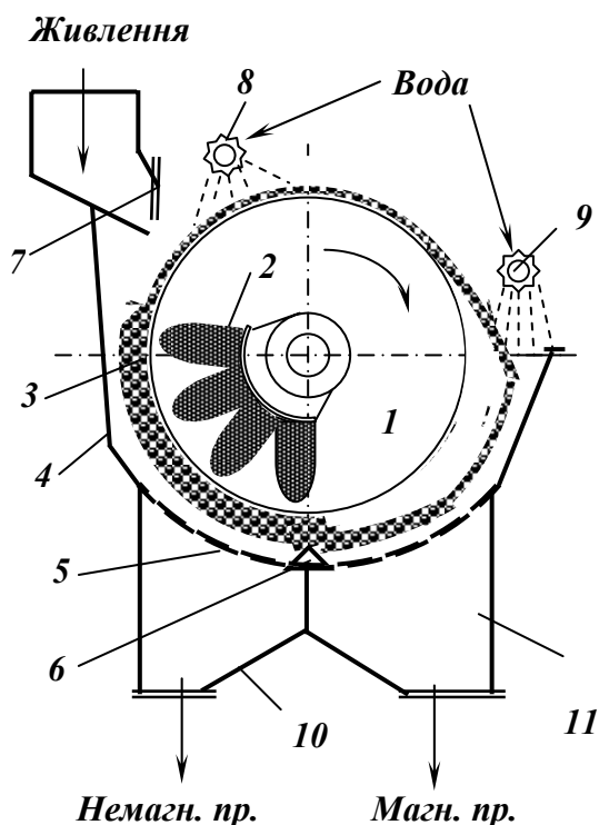
Рис. 7.14 – Схема поліградієнтного сепаратора.
