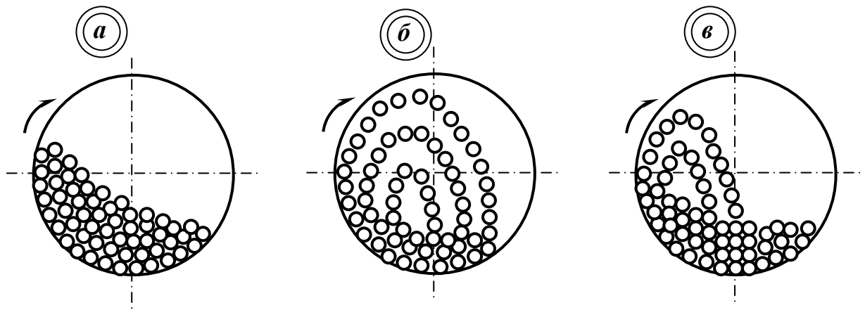
Рис. 4.41 – Режими роботи барабаних млинів. a – каскадний; б – водоспадний; в – змішаний.
