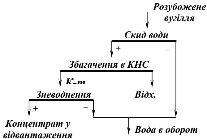
Рис. 5.44 – Схема збагачення розубоженого вугілля.
