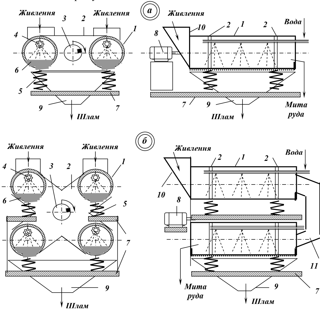
Рис. 4.62 – Схеми вібромилок.
