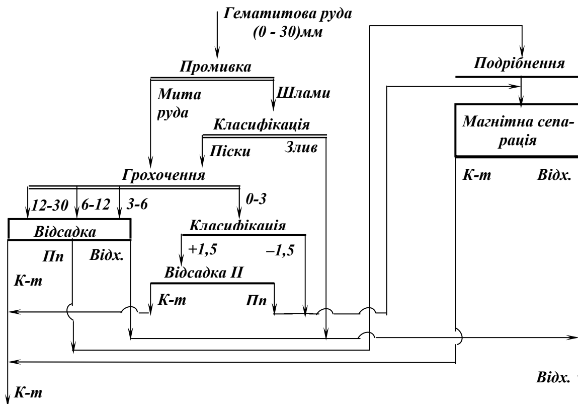
Рис. 7.20 – Схема збагачення гематитової руди відсадкою і магнітною сепарацією.
