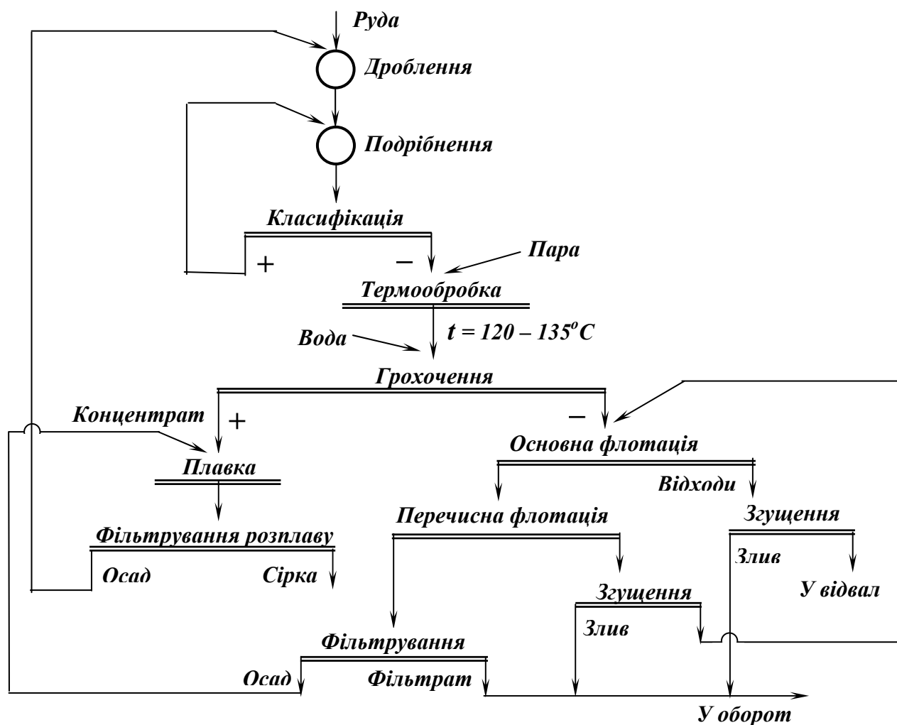
Рис. 9.35 – Комбінована схема переробки тонковкрапленої сірчаної руди.
