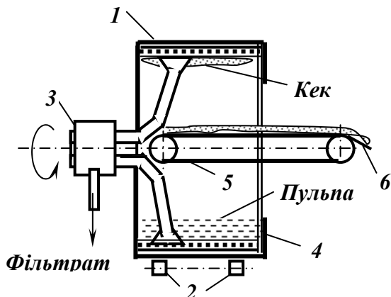
Рис. 10.15 – Схема барабанного вакуум-фільтра з внутрішньою фільтруючою поверхнею.
