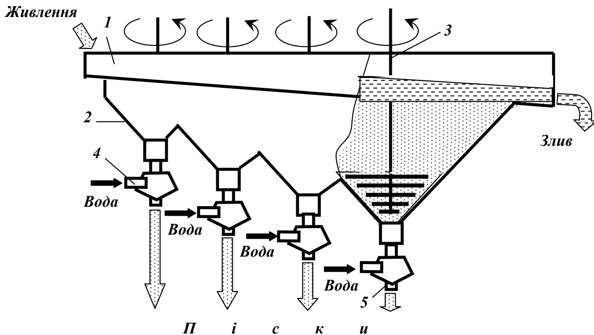
Рис. 4.54 – Гідралічний багатоканальний класифікатор.
