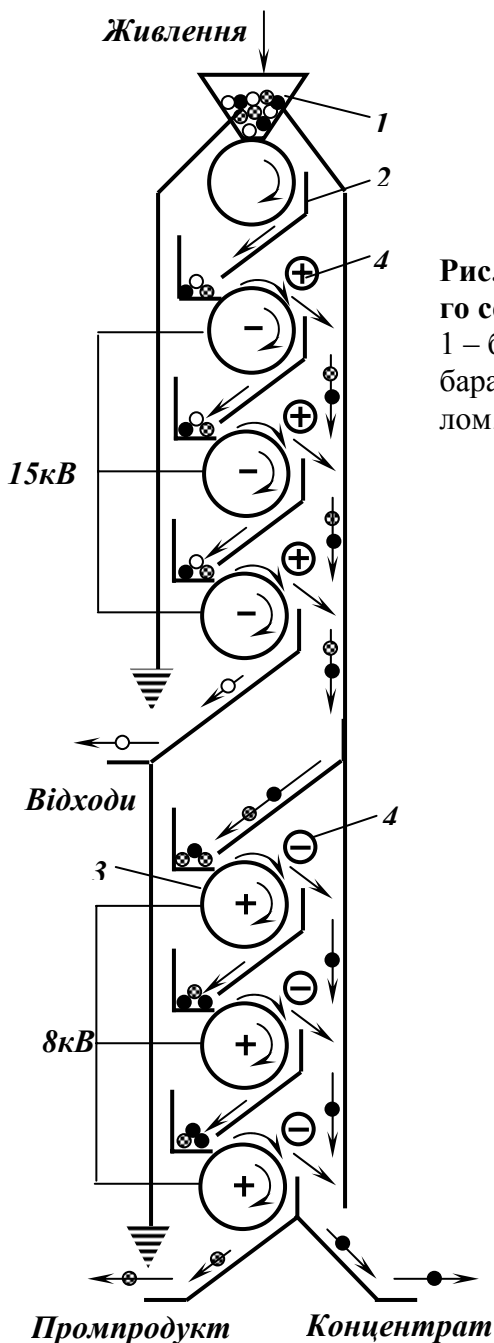
Рис. 8.9 – Трибоадгезійний сепаратор.
