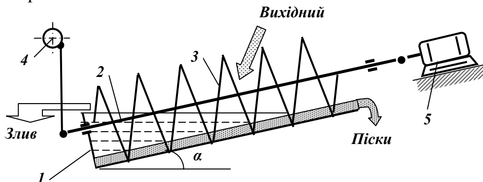
Рис. 4.48 – Спіральний класифікатор.
