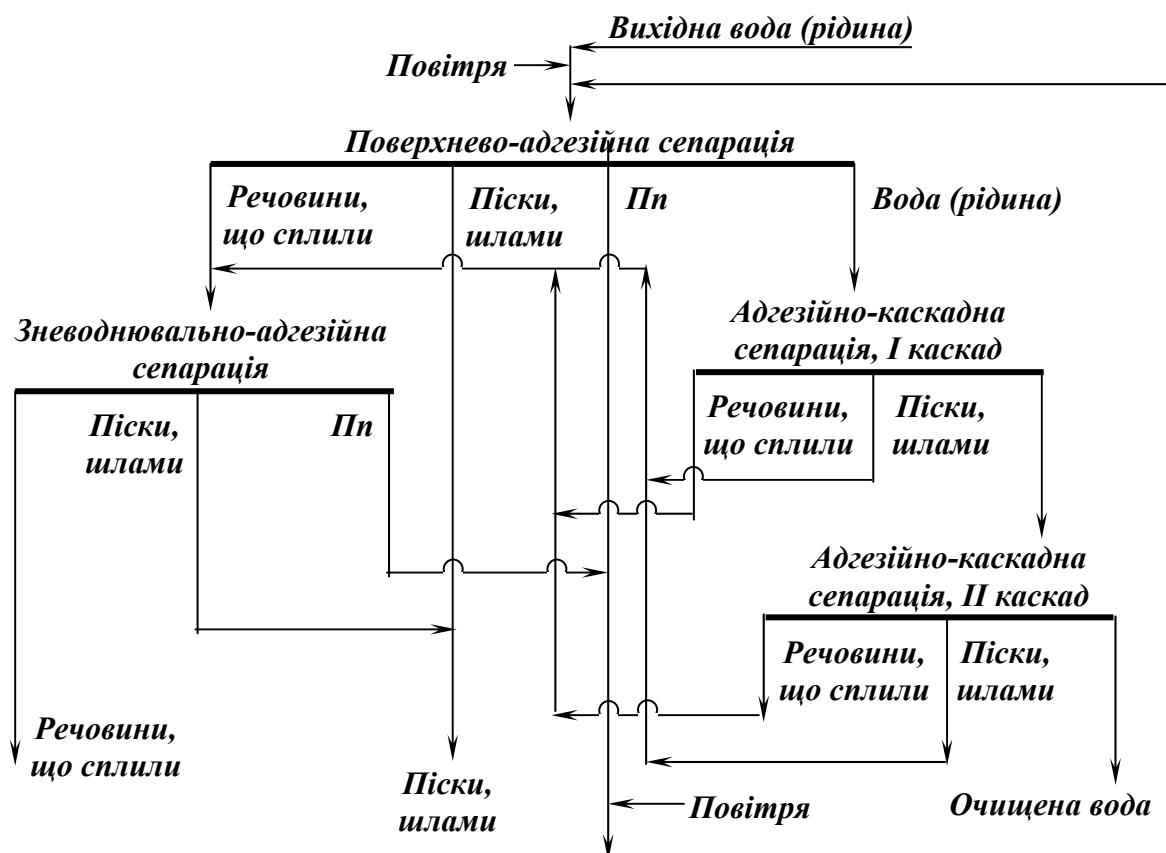
Рис. 12.7 – Схема пристрою поверхневої, каскадної і зневоднювальної адгезійної сепарації.
