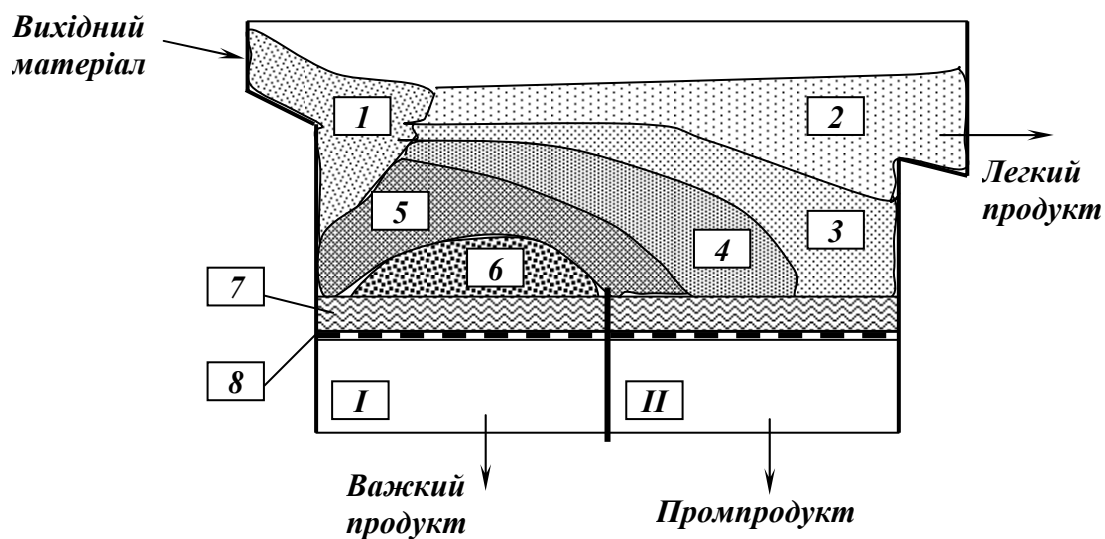
Рис. 5.17 - Розподіл продуктів у відсаджувальній машині.
