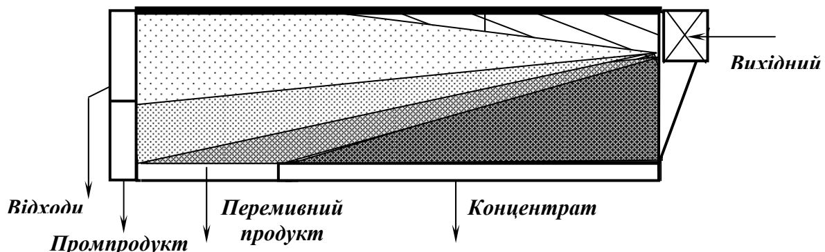
Рис. 5.48 – Схема розподілу продуктів на деці пневматичного сепаратора.
