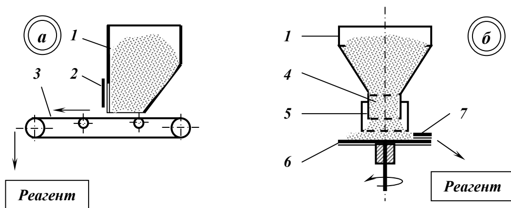
Рис. 6.16 – Схеми живильників для сипких реагентів. a – стрічковий; б – тарілчастий.
