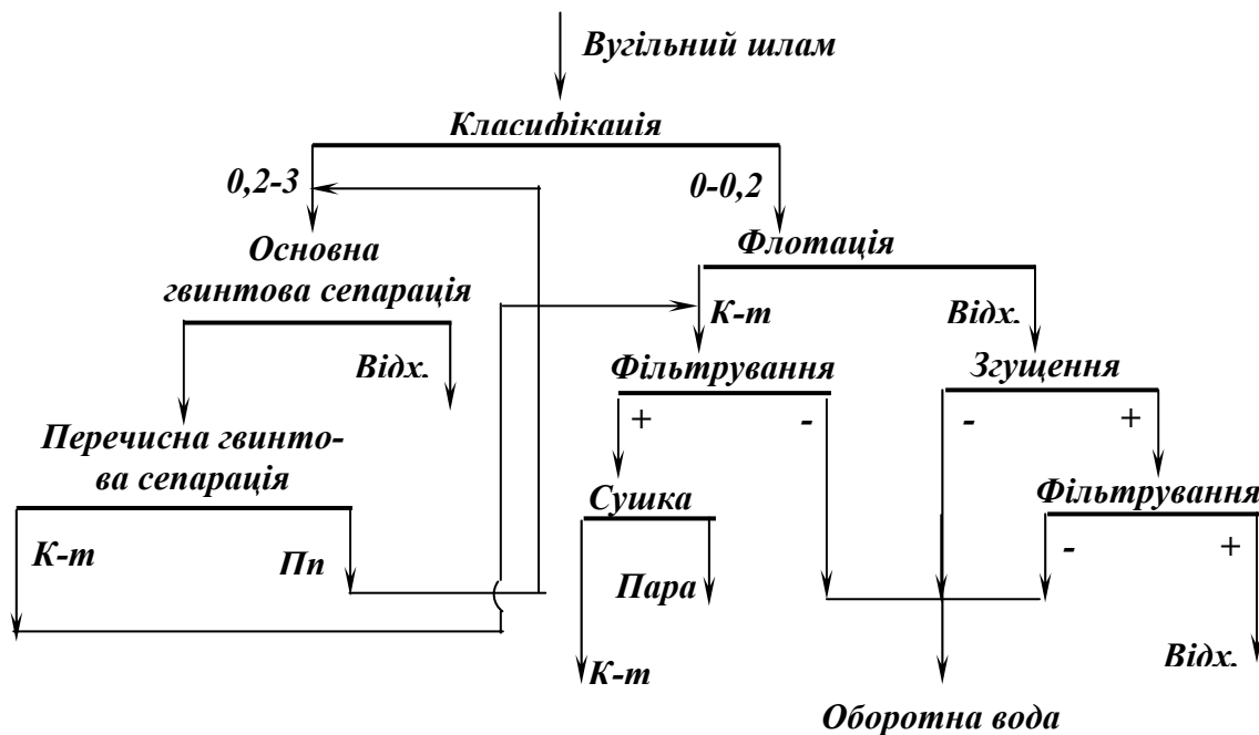
Рис. 6.27 – Схема збагачення вугільних шламів гвинтовою сепарацією і флотацією.
