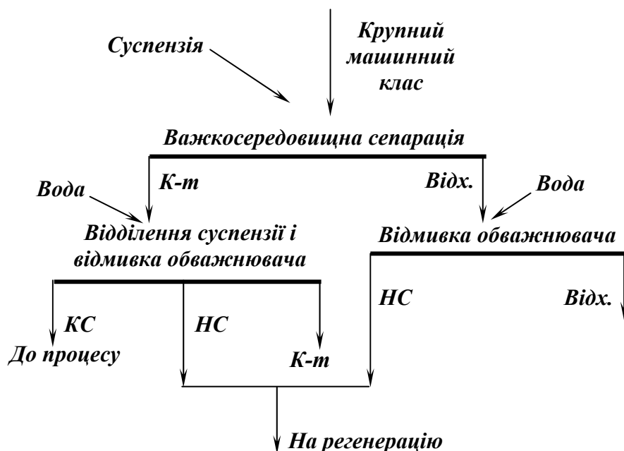
Рис. 5.10 – Схема важкосередовищної сепарації вугілля крупних класів у одну стадію з виділенням двох продуктів.
