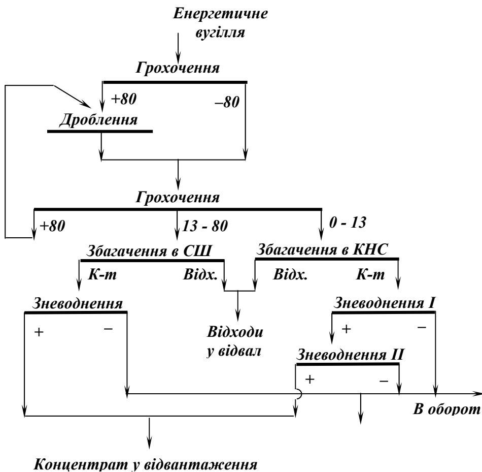
Рис. 5.46 – Схема збагачення енергетичного вугілля.
