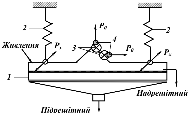
Рис. 4.15 – Схема інерційно-самобалансного грохота.
