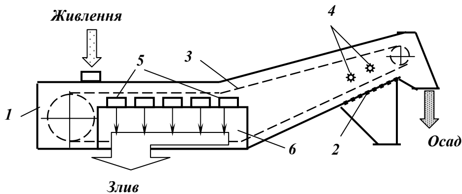
Рис. 4.51 - Скребковий класифікатор.
