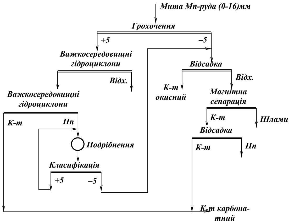
Рис. 7.23 – Схема переробки карбонатної марганцевої руди.
