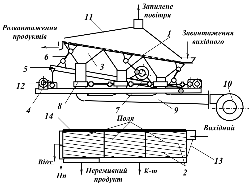
Рис. 5.47 – Схема повітряного сепаратора.
