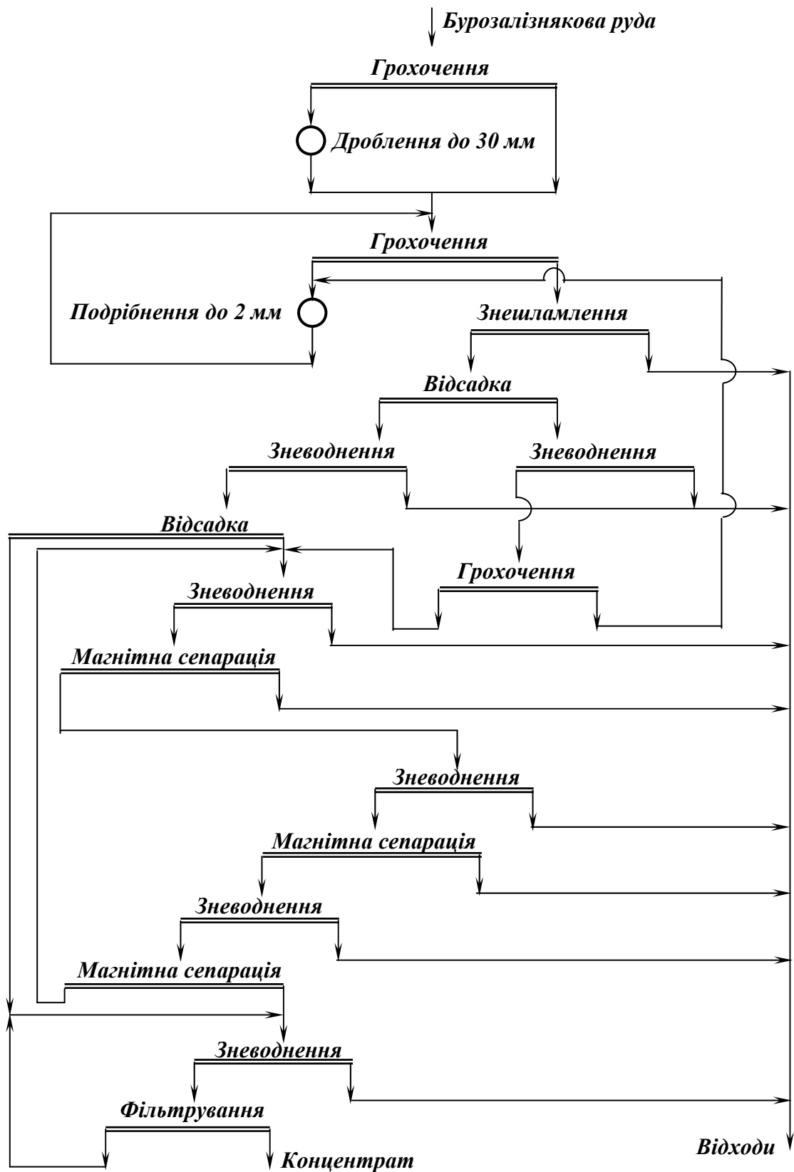
Рис. 7.21 – Схема збагачення бурозалізнякової руди.
