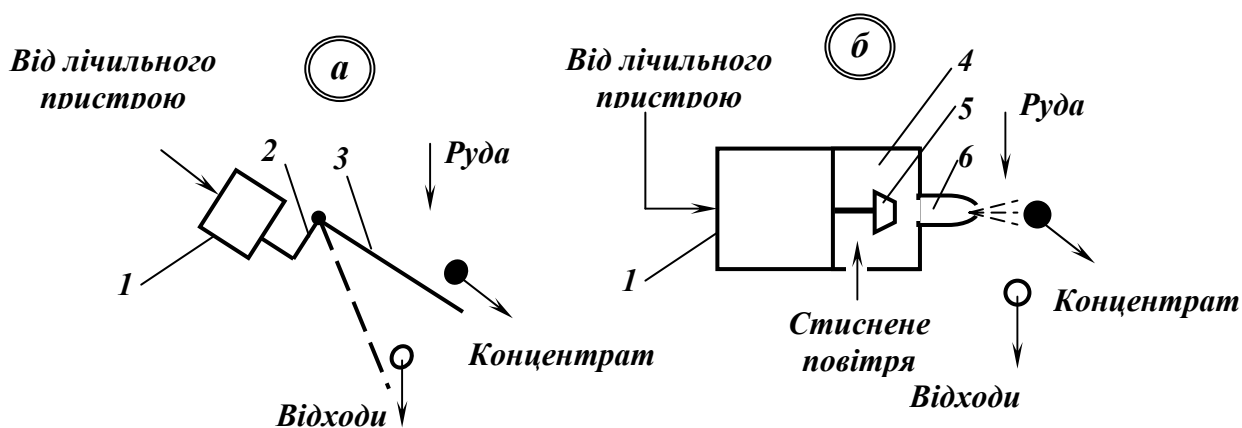
Рис. 9.10 – Виконавчі механізми.
