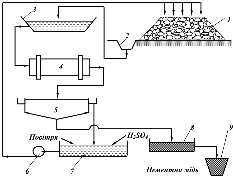
Рис. 9.37 – Схема кучного вилюговування мідної руди.
