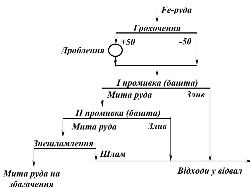
Рис. 4.51 – Схема промивки валунчатої лимонітової руди.
