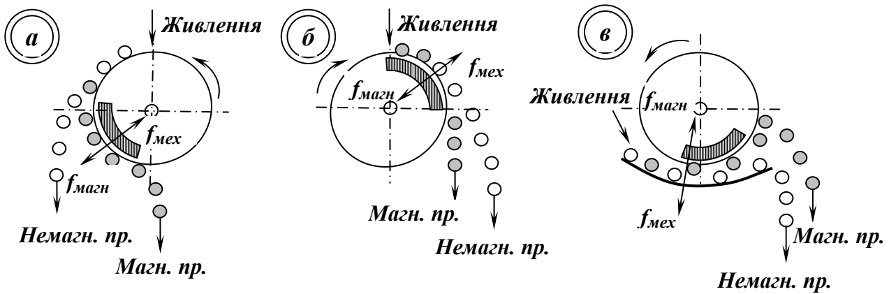
Рис 7.3 – Режими розділення частинок при магнітній сепарації. а – відхилення; б – утримання; в – вилучення.
