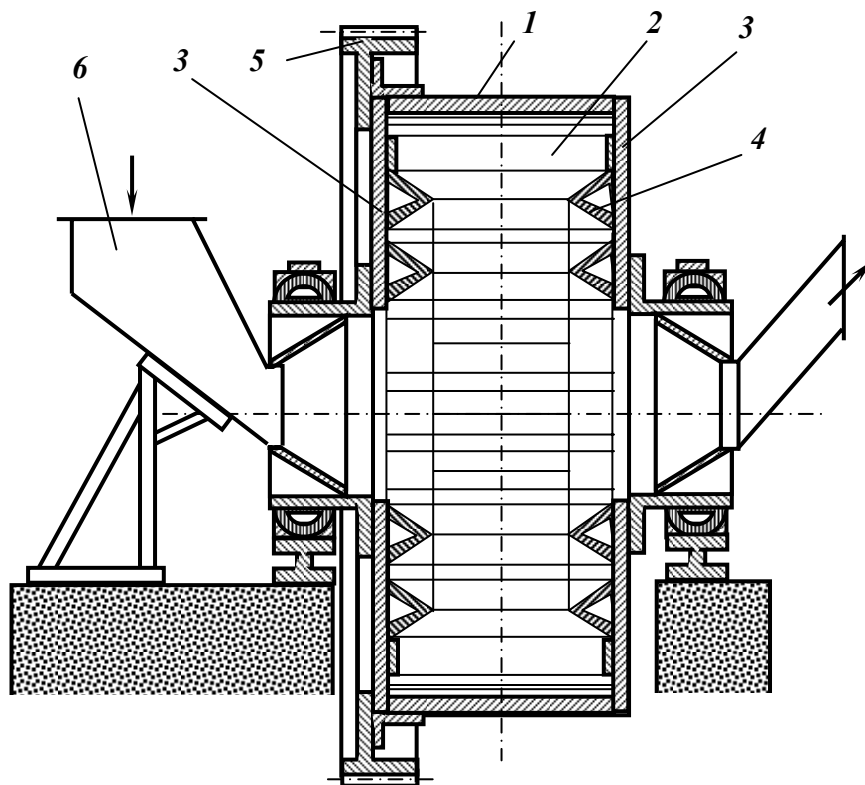
Рис. 4.45 – Млин сухого самоподрібнення типу «Аерофол».
