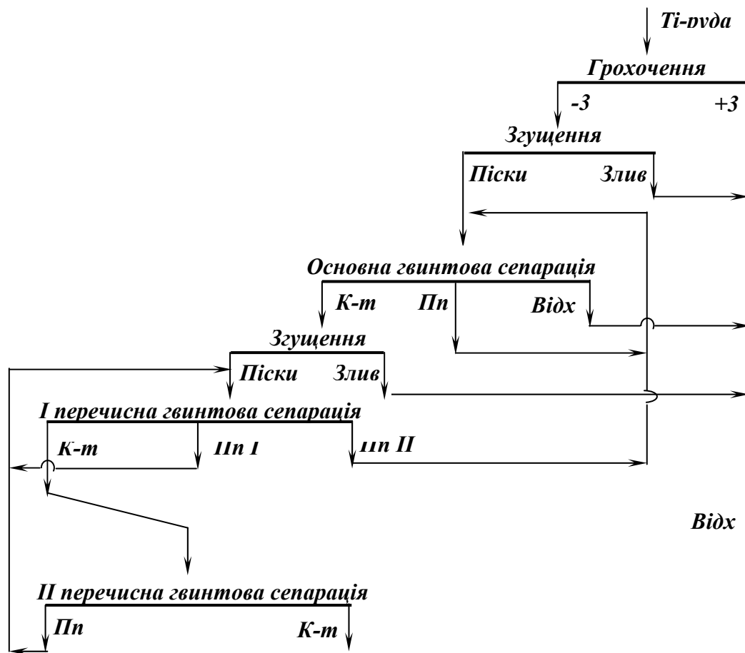
Рис. 5.38 – Схема збагачення титановмісної розсипної руди з використанням гвинтової сепарації.
