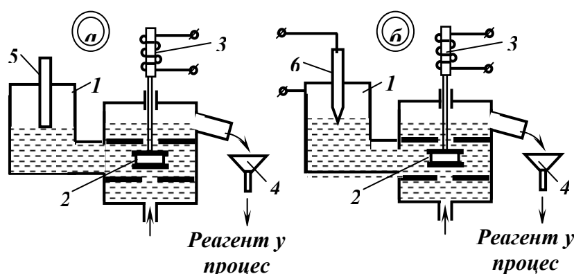
Рис. 6.22 – Схеми порційних живильників.
