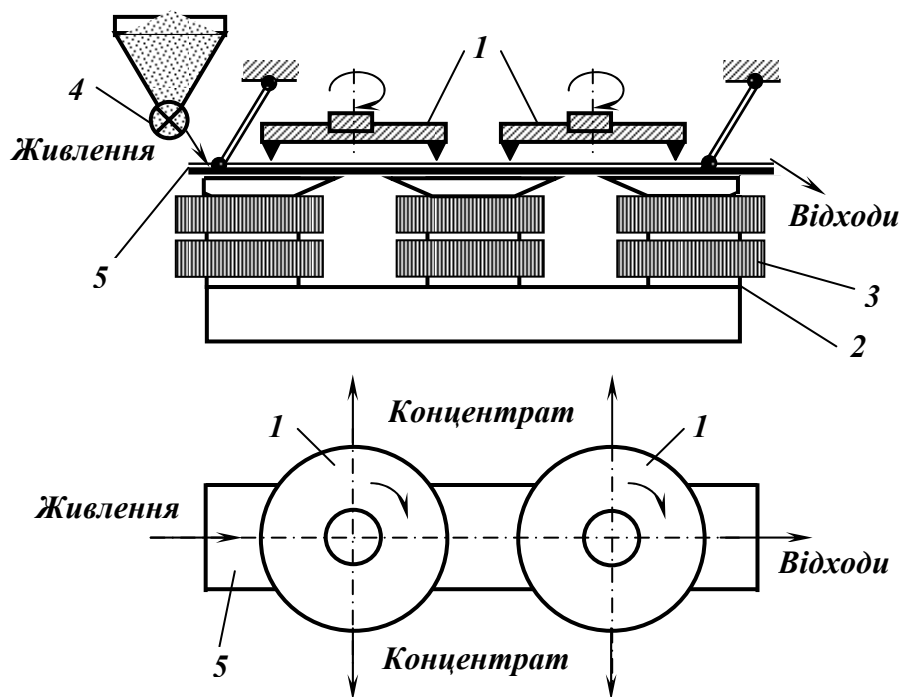
Рис. 7.13 – Схема дискового магнітного сепаратора.
