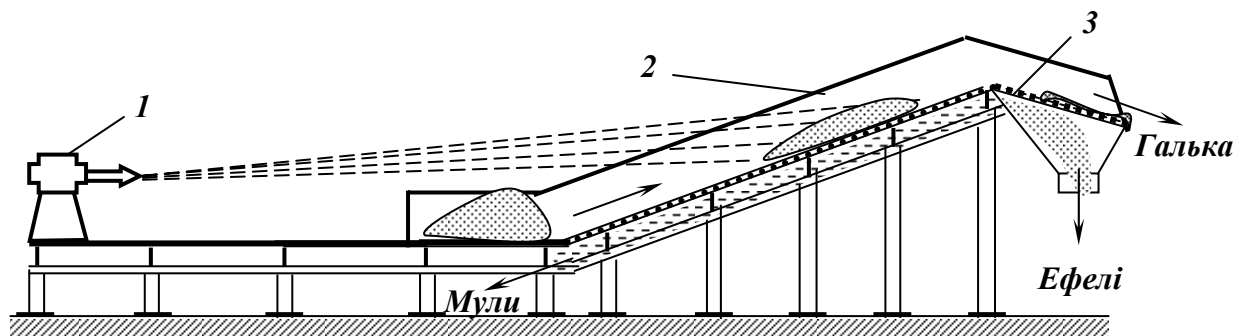
Рис. 4.57 – Схема гідравлічного вашгерда.
