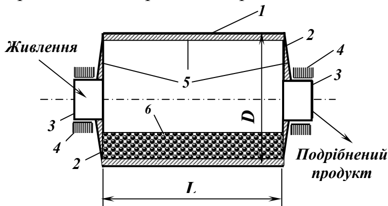
Рис. 4.40 – Схема барабанного млина.
