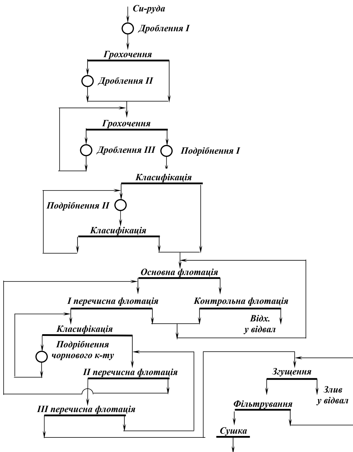
Рис. 6.28 – Технологічна схема збагачення вкраплених мідних руд.
