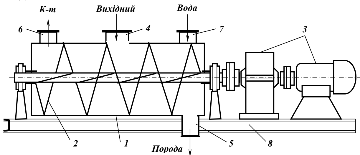
Рис. 5.40 – Схема горизонтального шнекового сепаратора.
