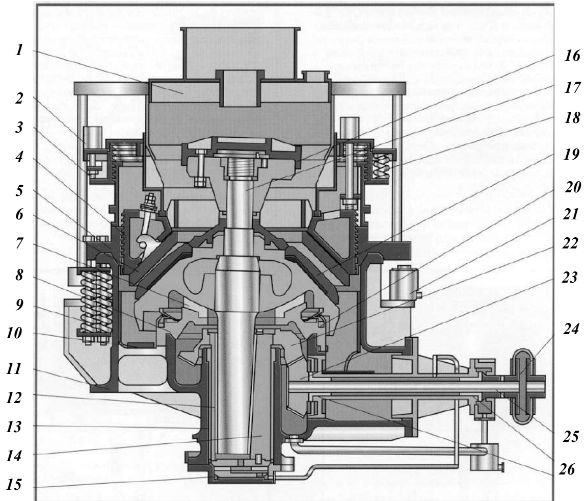
Рис. 4.28 – Конусна дробарка типу КМД-2200Г.
