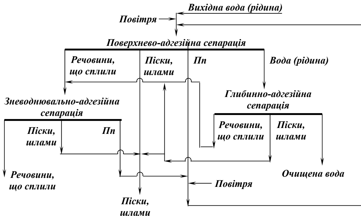
Рис. 12.8 – Схема пристрою поверхневої, глибинної і зневоднювальної адгезійної сепарації.
