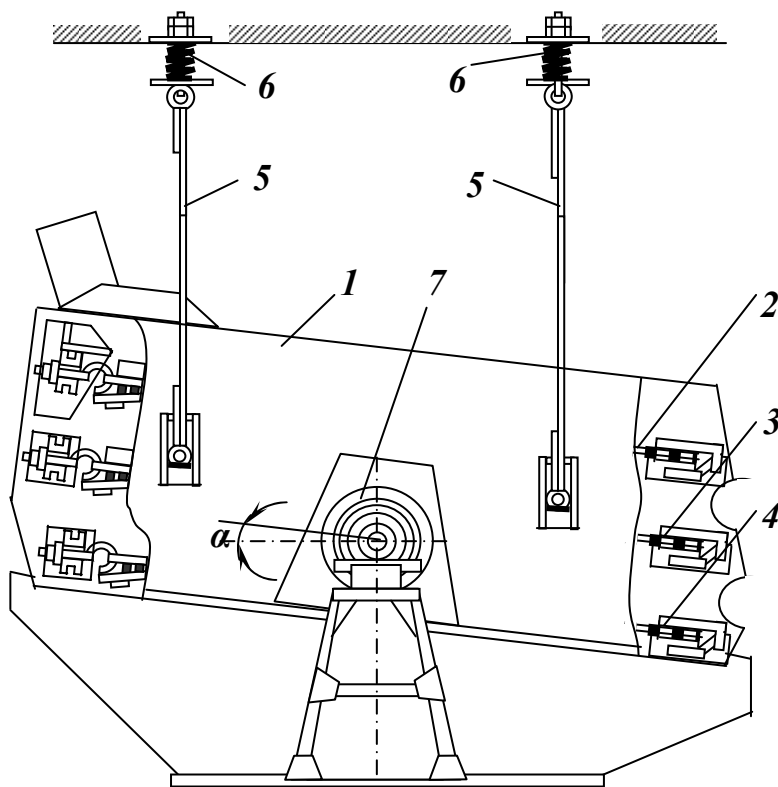
Рис. 4.14 – Грохот ГІЛ-43 в підвісному виконанні.
