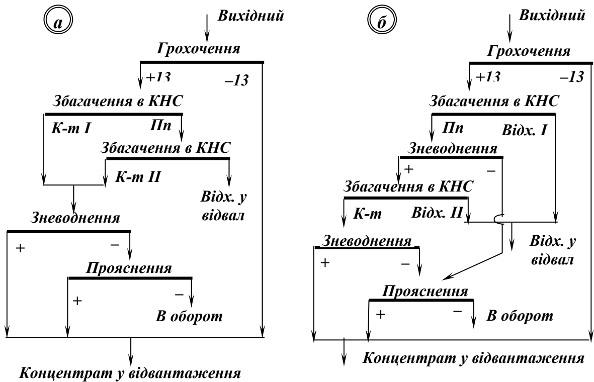
Рис. 4.46 – Двостадійні схеми збагачення вугілля в КНС.
