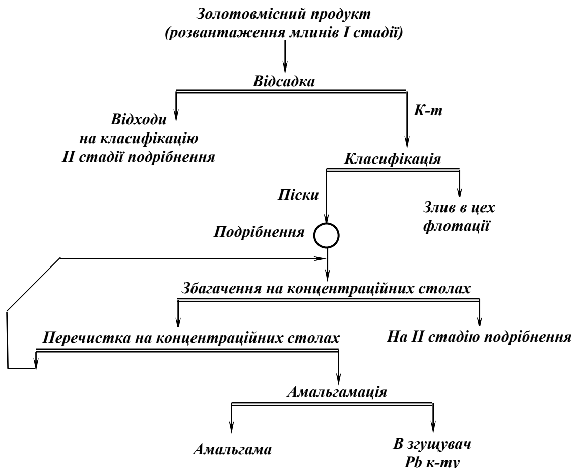
Рис. 11.7 – Технологічна схема збагачення секції вилучення золота.
