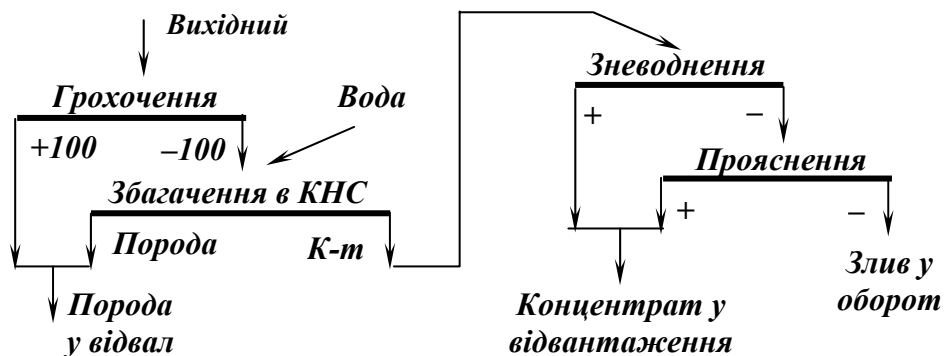
Рис. 5.43 – Схема вилучення горючої маси з відвальної породи.
