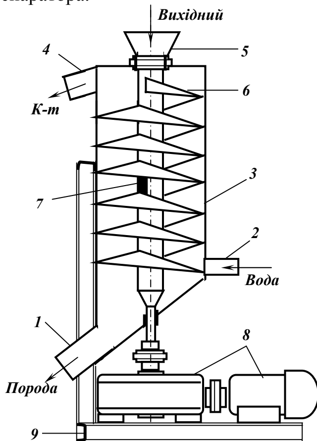
Рис. 5.41 – Схема вертикального шнекового сепаратора.
