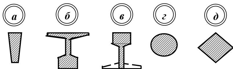
Рис. 4.6 – Профілі колосників.
