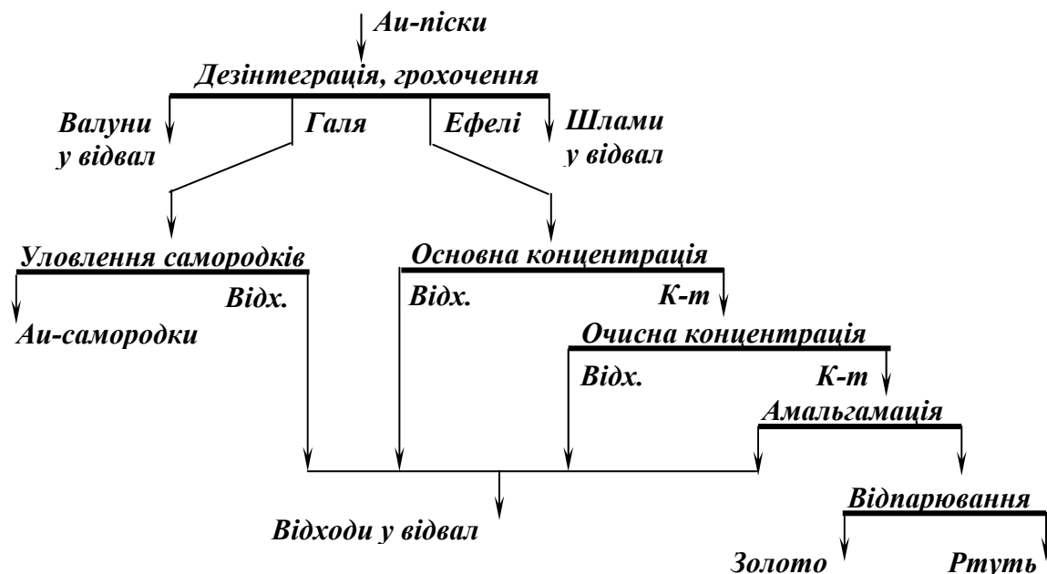
Рис. 4.52 – Типова схема збагачення золотовмісних пісків.
