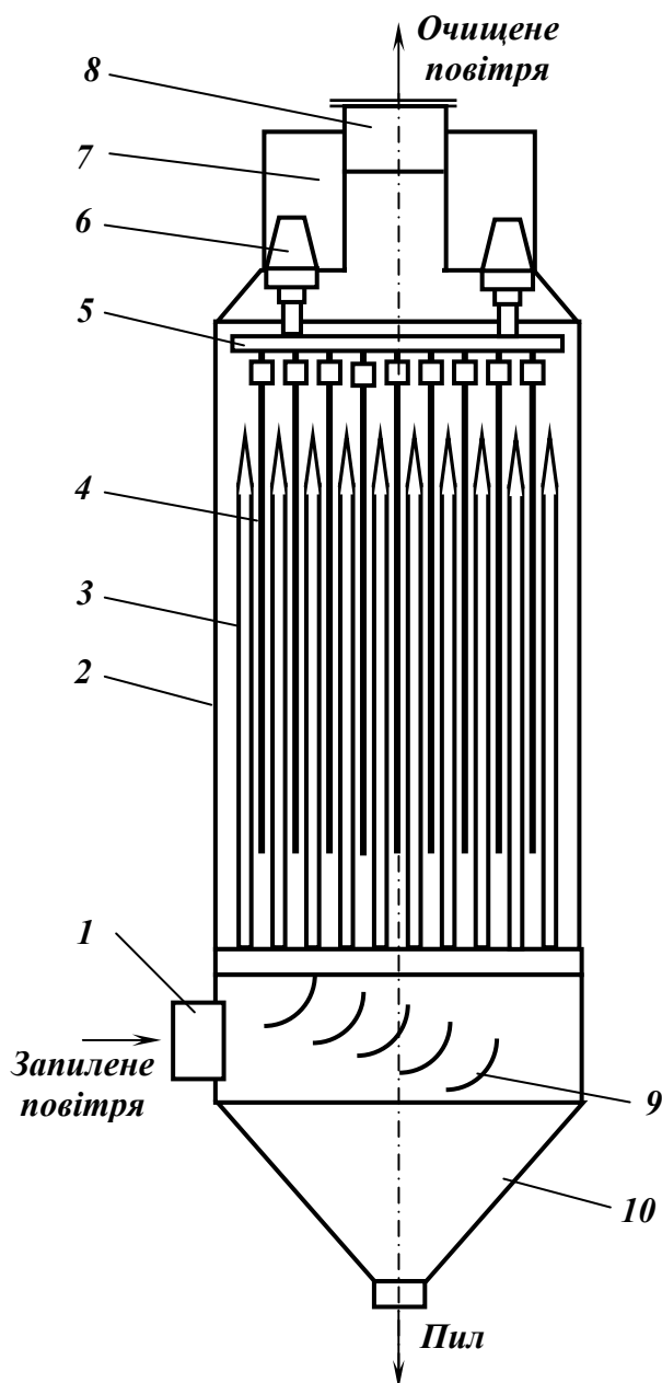
Рис. 10.37 – Електрофільтр ДВП.
