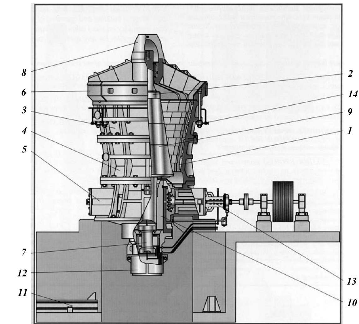
Рис. 4.25 – Конусна дробарка з гідравлічним регулюванням вихідної щілини типу ККД.
