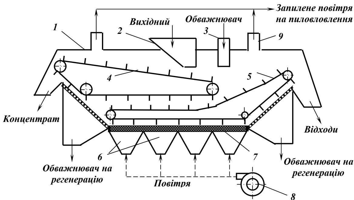
Рис. 5.50 – Схема аеросуспензійного сепаратора.
