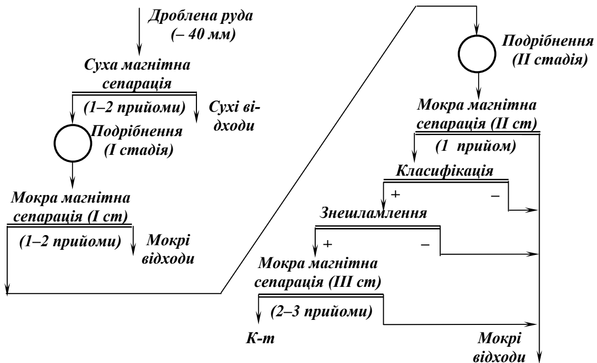
Рис. 7.16 – Схема магнітного збагачення скарнової магнетитової руди.
