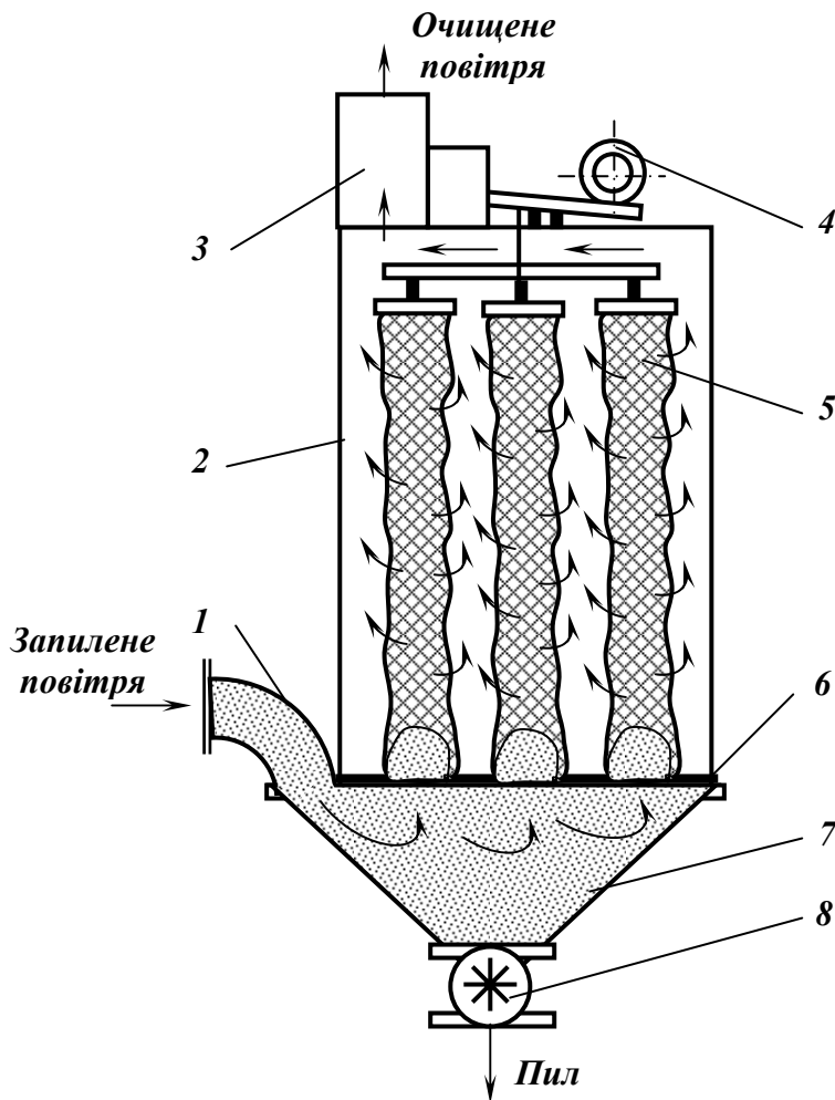
Рис. 10.33 – Рукавний фільтр.
