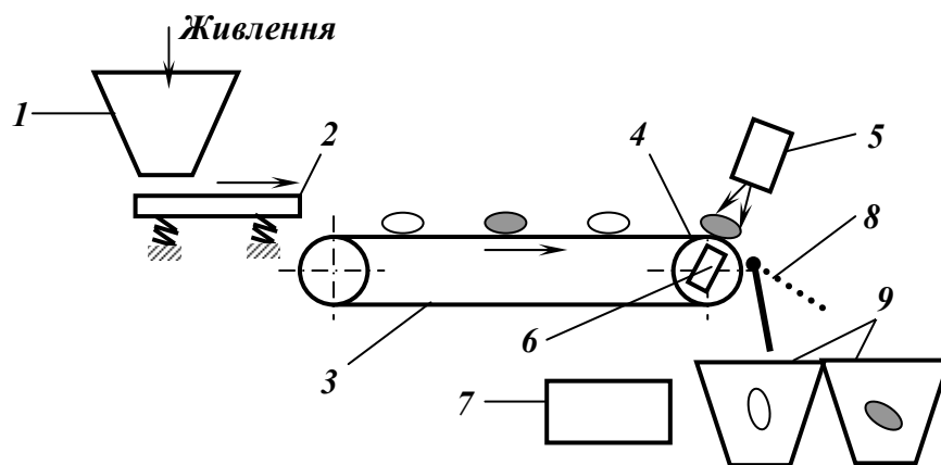
Рис. 9.16 – Схема гамма-абсорбційного сепаратора.
