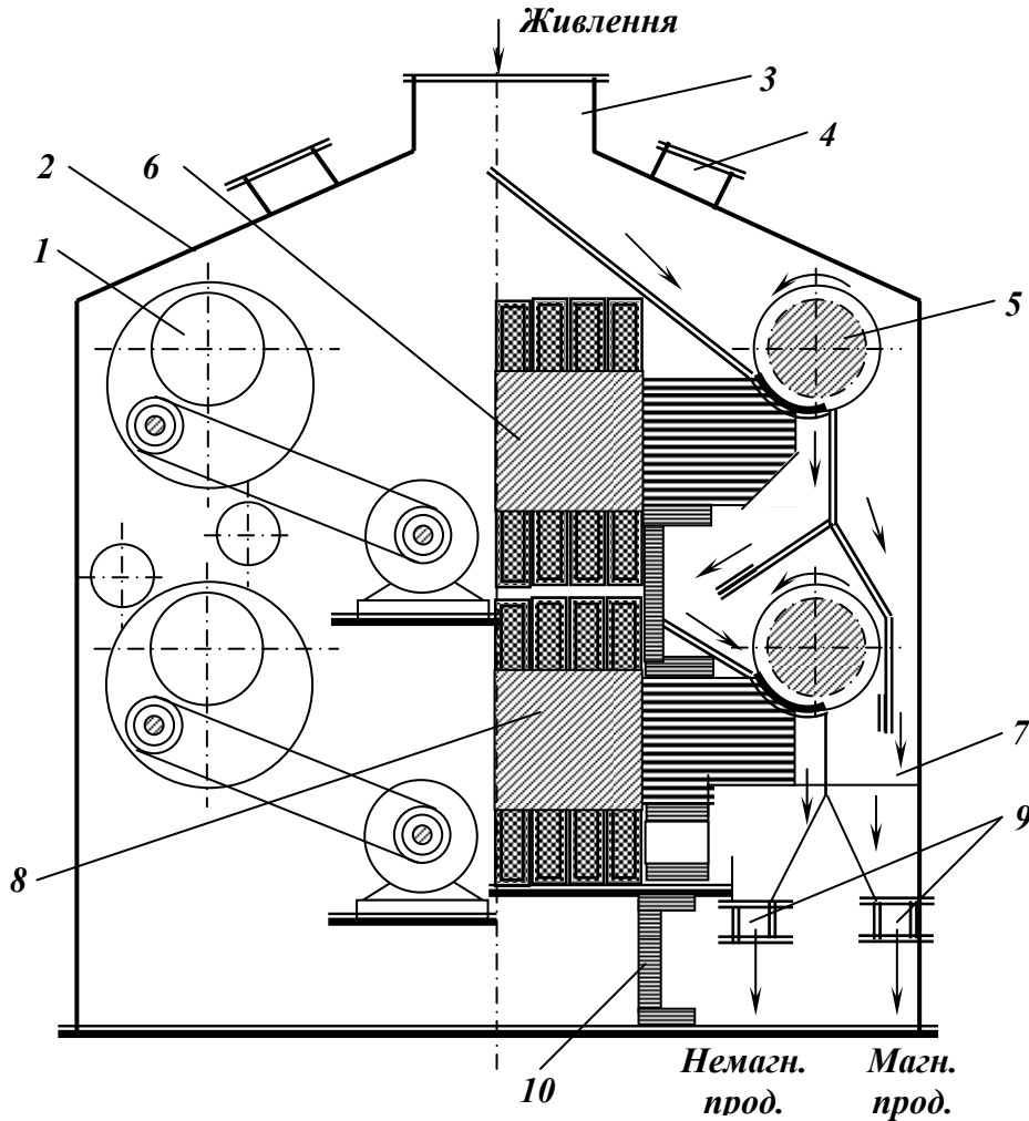
Рис. 7.12 – Схема електромагнітного валкового сепаратора типу 8ЕВС-16/100.
