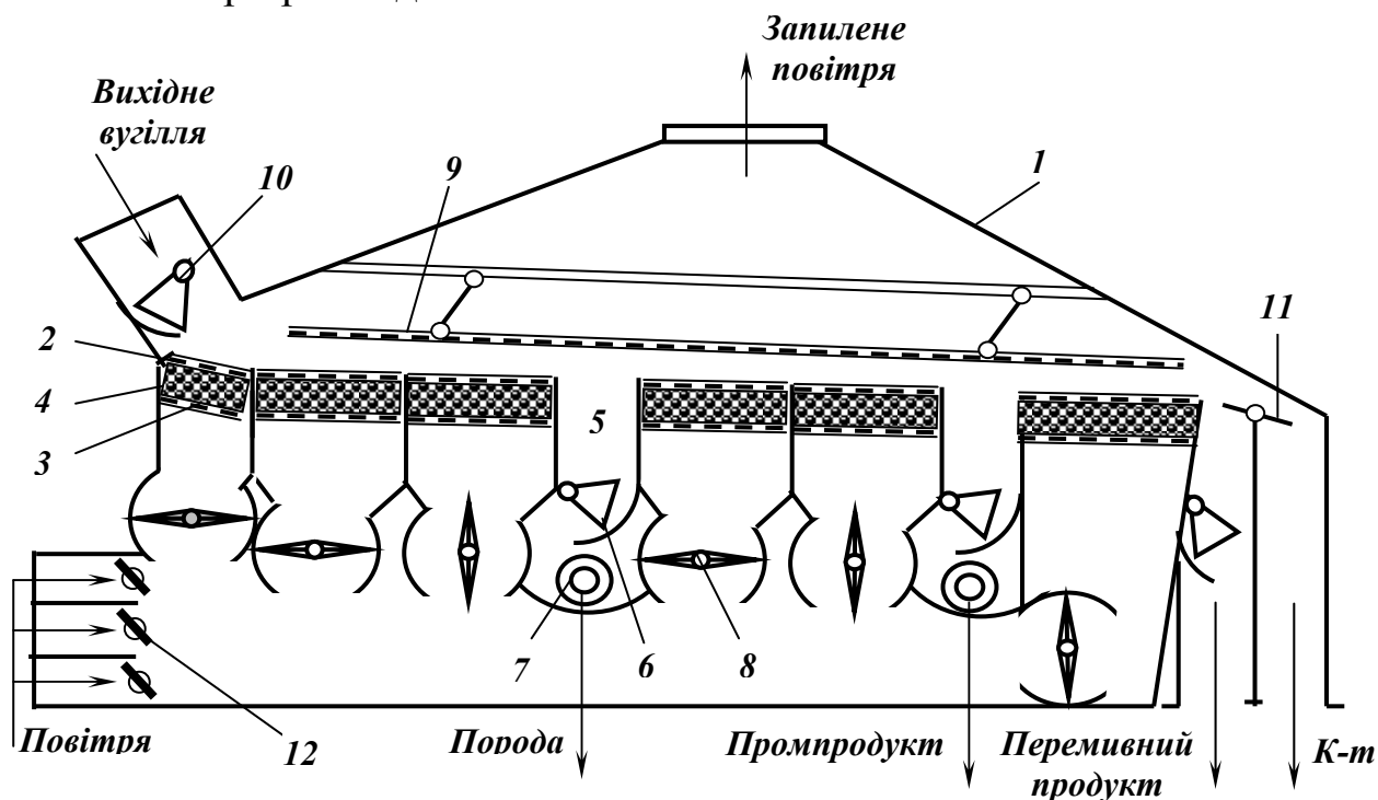
Рис. 5.49 – Схема повітряної відсаджувальної машини.
