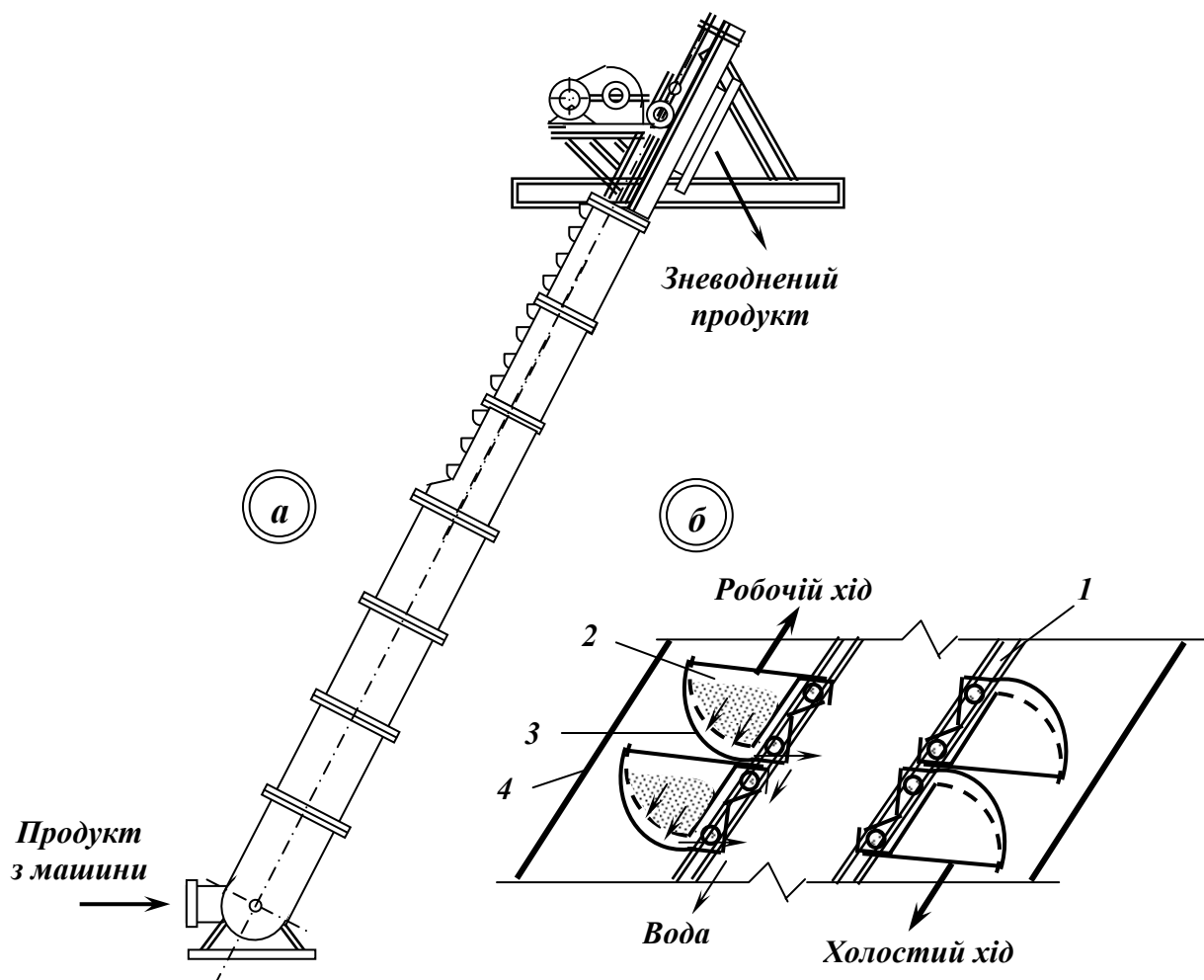
Рис. 10.3 – Зневоднювальний елеватор.
