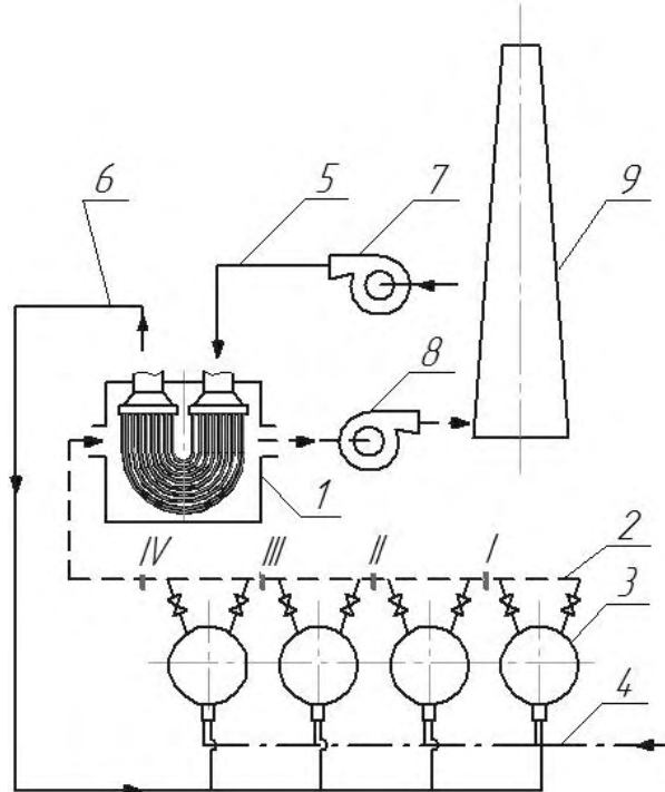
Рис. 2 – Спрощена схема утилізації теплоти димових газів блоку регенеративних доменних повітрянагрівачів:
