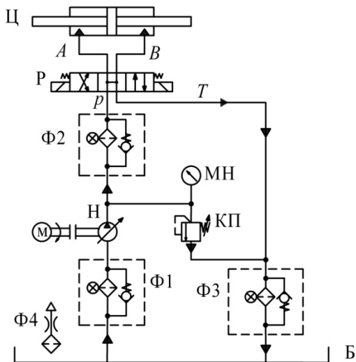
Рис. 1 – Типові місця встановлення фільтрів в об'ємному гідروприводі: Н – насос з регульованим робочим об'ємом; «М» – електродвигун; Ц – гідроциліндр; Р – гідророзподільник; КП – клапан запобіжний; Б – гідробак; МН – манометр; Ф1; Ф2 і Ф3 – фільтри для очищення РР; Ф4 – повітряний фільтр (сапун).
