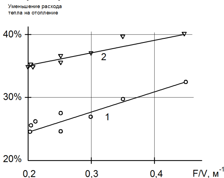
Рисунок. Сравнение эффективности утепления зданий: 1 – при дополнительном утеплении наружных ограждений 2 – при утеплении ограждений и энергосбережении в системе вентиляции
