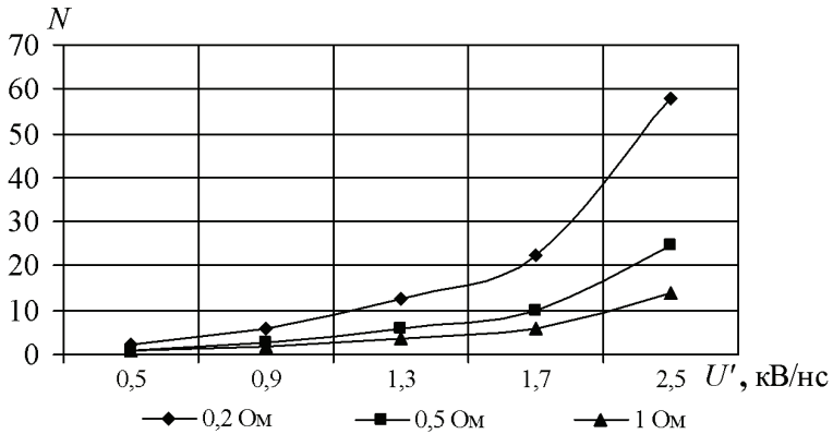
Рисунок 2 – Зависимость числа параллельных каналов N от скорости нарастания амплитуды управляющего импульса U' для различных сопротивлений разрядного контура Z ( E = 3,354 кВ/мм)
