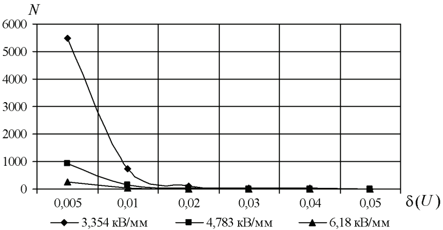
Рисунок 4 – Зависимость числа параллельных каналов N от величины относительного разброса \delta(U) напряжения срабатывания каналов для различных значений пробивной напряженности E ( U = 1,12 кВ/нс)
