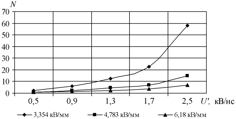
Рисунок 3 – Зависимость числа параллельных каналов N от скорости нарастания амплитуды управляющего импульса U' для различных значений пробивной напряженности E ( Z = 0,2 Ом)
