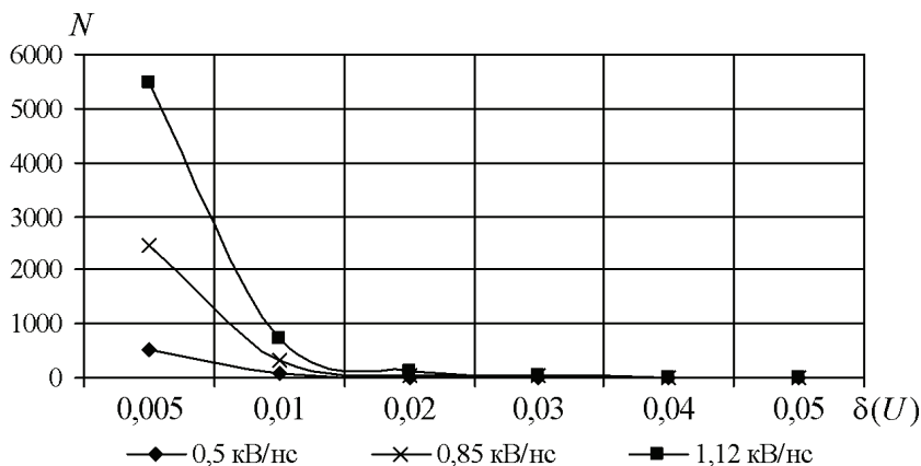
Рисунок 5 – Зависимость числа параллельных каналов N от величины относительного разброса \delta(U) напряжения срабатывания каналов для различных значений скорости нарастания амплитуды управляющего импульса U' ( E=3,354 кВ/мм)
