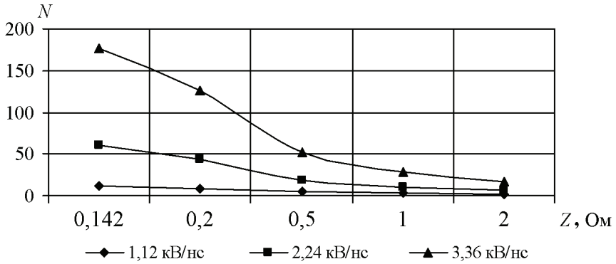
Рисунок 1 – Зависимость числа параллельных каналов N от сопротивления разрядного контура Z для различных значений скорости нарастания амплитуды управляющего импульса ( E=3,354 кВ/мм)
