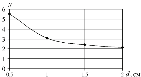
Рисунок 6 – Зависимость числа параллельных каналов N от длины разрядного промежутка d
