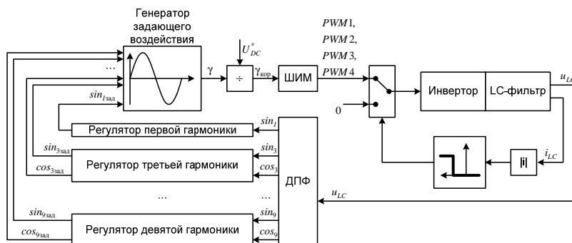
Рис. 2. Функциональная схема структуры системы управления
