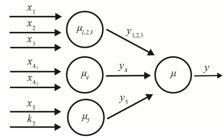
Рис. – Схема модели качества пространственных данных
