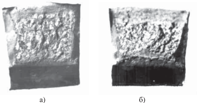
Рис. 3. Поверхность излома ударных образцов с V-образным надрезом посередине металла шва: \times 5,5 . а) – автоматическая сварка по штатной технологии; б) – по предлагаемой
