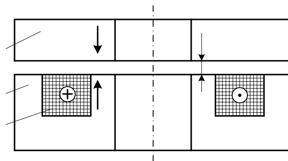
Рис. 1. Магнитная система электромагнитного линейного импульсного электродвигателя
