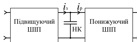
Рис. 4. Структура, яка підтримує рівність струмів
