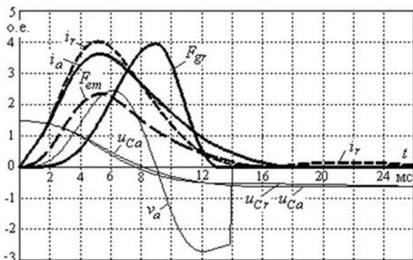
Рис. 7. Временные функции величин при независимом питании обмоток
