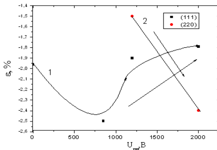
Рис. 6. Залежність макродеформації кристалічної решітки покриттів нітриду титану, отриманих при U_{\text{прі}} = -200 В в залежності від величини U_{\text{прі}} .
