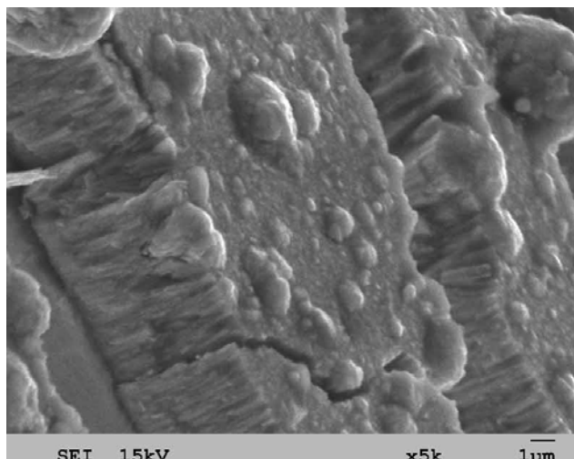
Рис. 3. Морфологія зламу TiN покриття. U_{\min} = (-5 \dots -8) В, U_{\text{пл}} = -1 кВ, f = 7 кГц.
