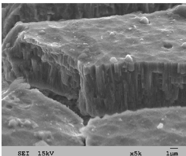
Рис. 2. Морфологія зламу TiN покриття. U_{\min} = -200 В, U_{\text{пл}} = -1 кВ, f = 7 кГц.
