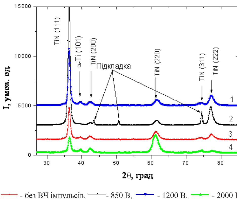
Рис. 5. Ділянки рентгендифракційних спектрів від покриттів нітриду титану, отриманих при U_{\text{прі}} = -200 В у випадках відсутності імпульсного високовольтного впливу (1), при U_{\text{прі}} = -850 В (2), при U_{\text{прі}} = -1200 В (3), при U_{\text{прі}} = -2000 В (4)
