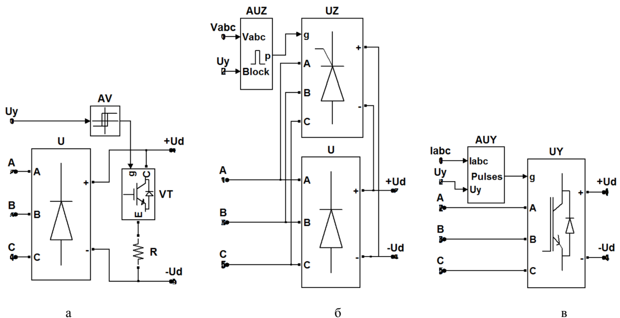
Рисунок 2 – Виртуальные модели тормозных модулей: а – тормозной резистор; б – дополнительная группа вентиляей; в – активный выпрямитель
