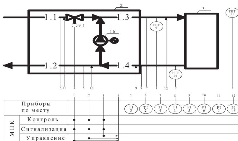
Рис. 2. Фрагмент ФСА ТП ФМИТП (2) и ФМСО (3), где 1.1 – горячий теплоноситель после ФМИТЭ (на схеме не показана); 1.2 – теплоноситель в ФМИТЭ; 1.3 – горячий смешанный теплоноситель после ФМИТП (в ФМСО); 1.4 – теплоноситель после ФМСО
