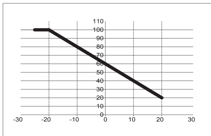
Рис. 3. Температурный график управления температурой горячего смешанного теплоносителя (Y) после ФМИТП (в ФМСО) с коррекцией по температуре наружного воздуха (X 1 ) как возмущающего воздействия
