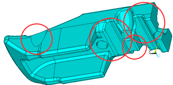
Рисунок 22 – Зони згущення сітки
