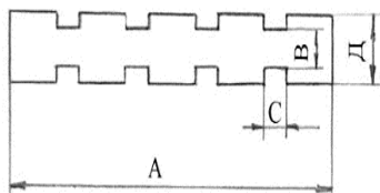
Рис. 2 – Плавкий елемент запобіжника типу GS на 1000В (амплітудне значення).
