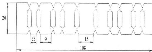
Рис. 4 – Плавкий елемент запобіжника LKNES.
