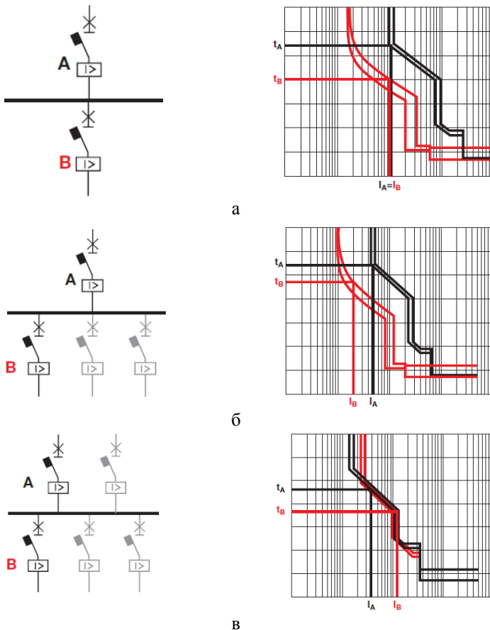
Рис. 4 – Часо-струмові характеристики увімкнених послідовно вимикачів: а – один автоматичний вимикач на боці живлення і один автоматичний вимикач на стороні навантаження; б – один автоматичний вимикач на боці живлення й кілька автоматичних вимикачів на стороні навантаження; в – два або більше автоматичних вимикачів на стороні живлення й кілька автоматичних вимикачів на стороні навантаження.
