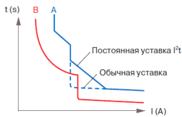
Рис. 22 – Логічна селективність апаратів Legrand.
