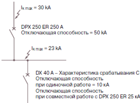
Рис. 16 – Координация работы выключателей Legrand.
