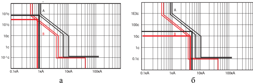
Рис. 5 – Захисні характеристики вимикачів при часострумовій селективності: а – автоматичний вимикач А з боку живлення спрацює за нижньою кривою; б – автоматичний вимикач з боку навантаження В спрацює за верхньою кривою.
