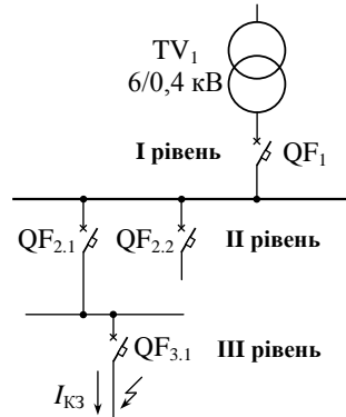
Рис. 17 – Координация в трёх уровнях.
