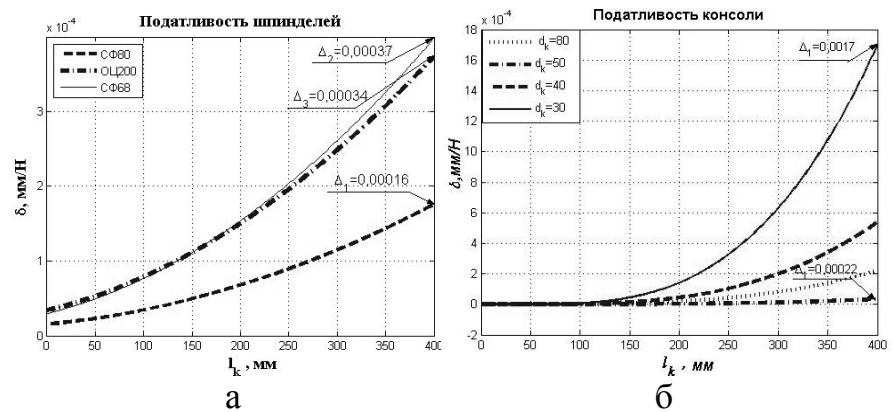
Рис.4 - Податливість шпиндельного узла: а – податливість шпинделя оброблюючого центра (статичний формуляр); б – податливість інструментального блоку (консоли)
